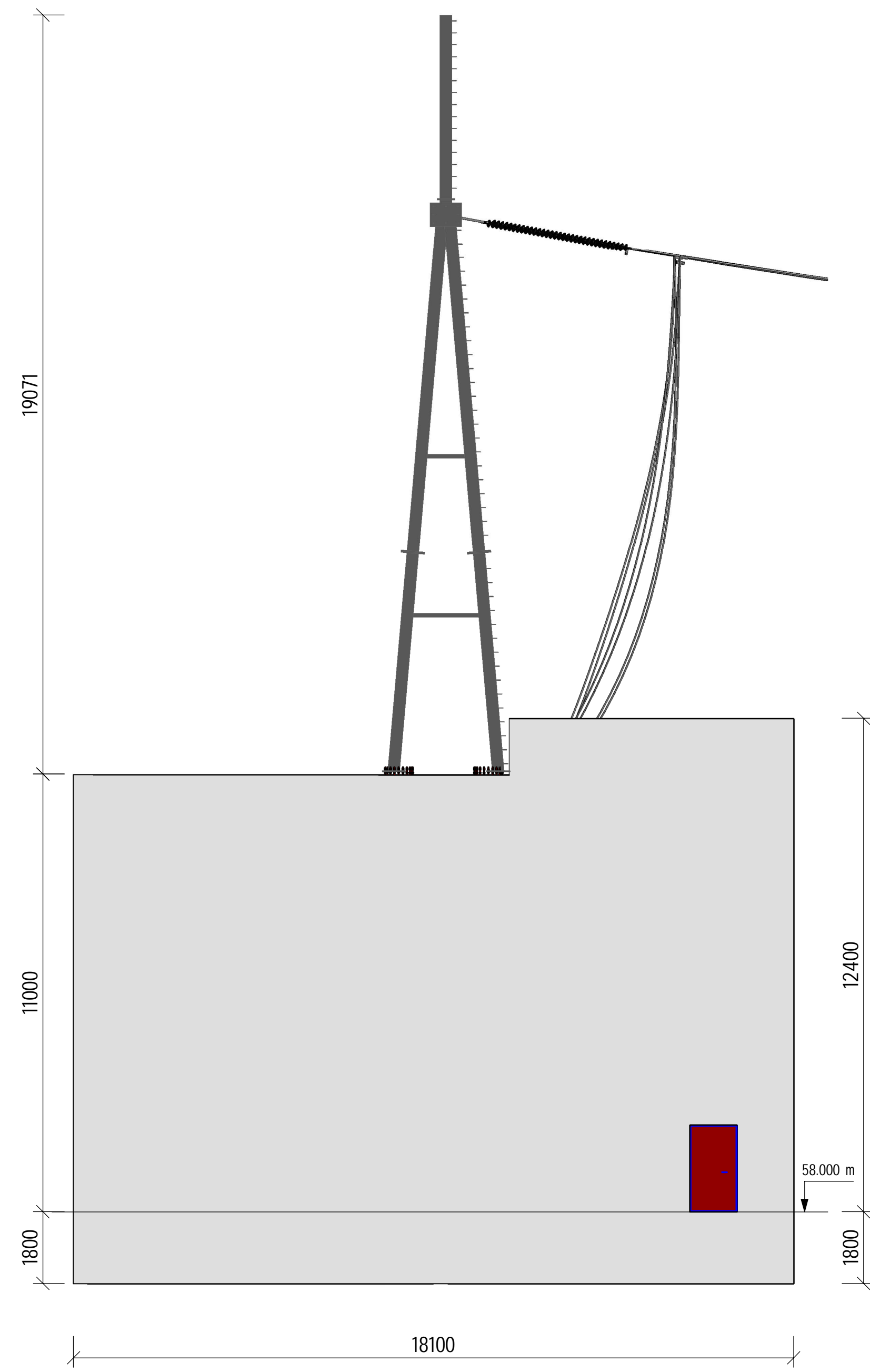
Fasade vest 1 : 100
