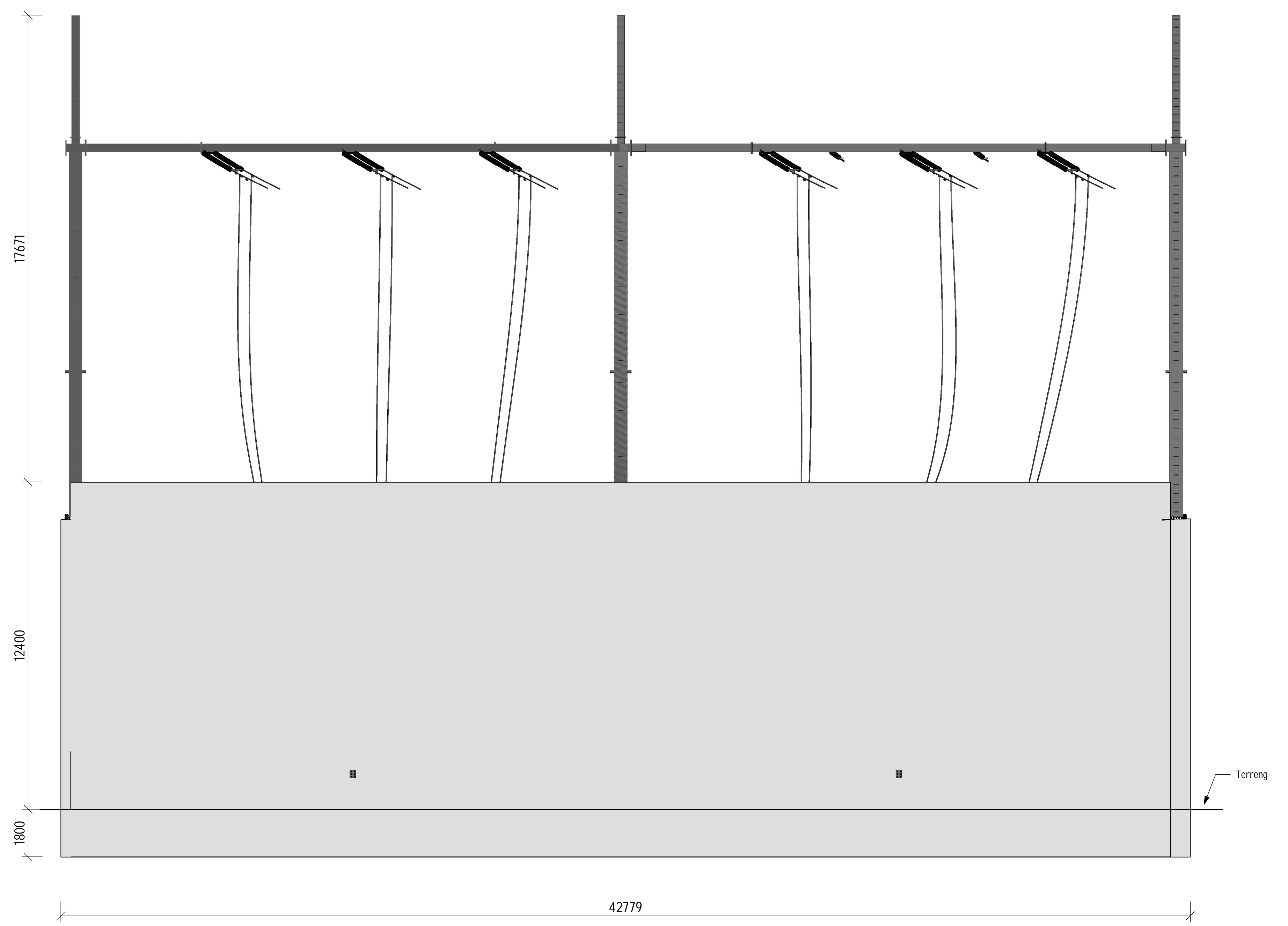
Fasade sør 1 : 100
