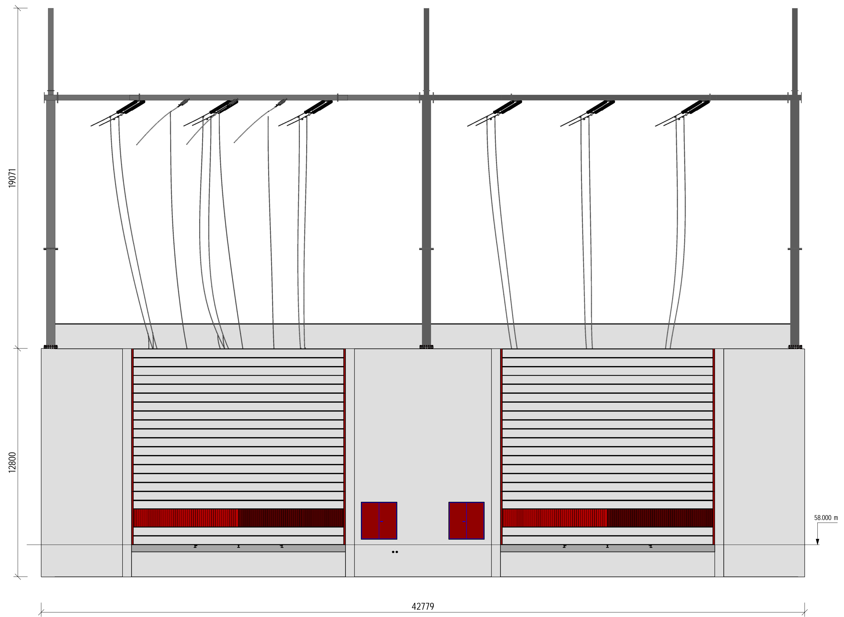
Fasade nord 1 : 100
