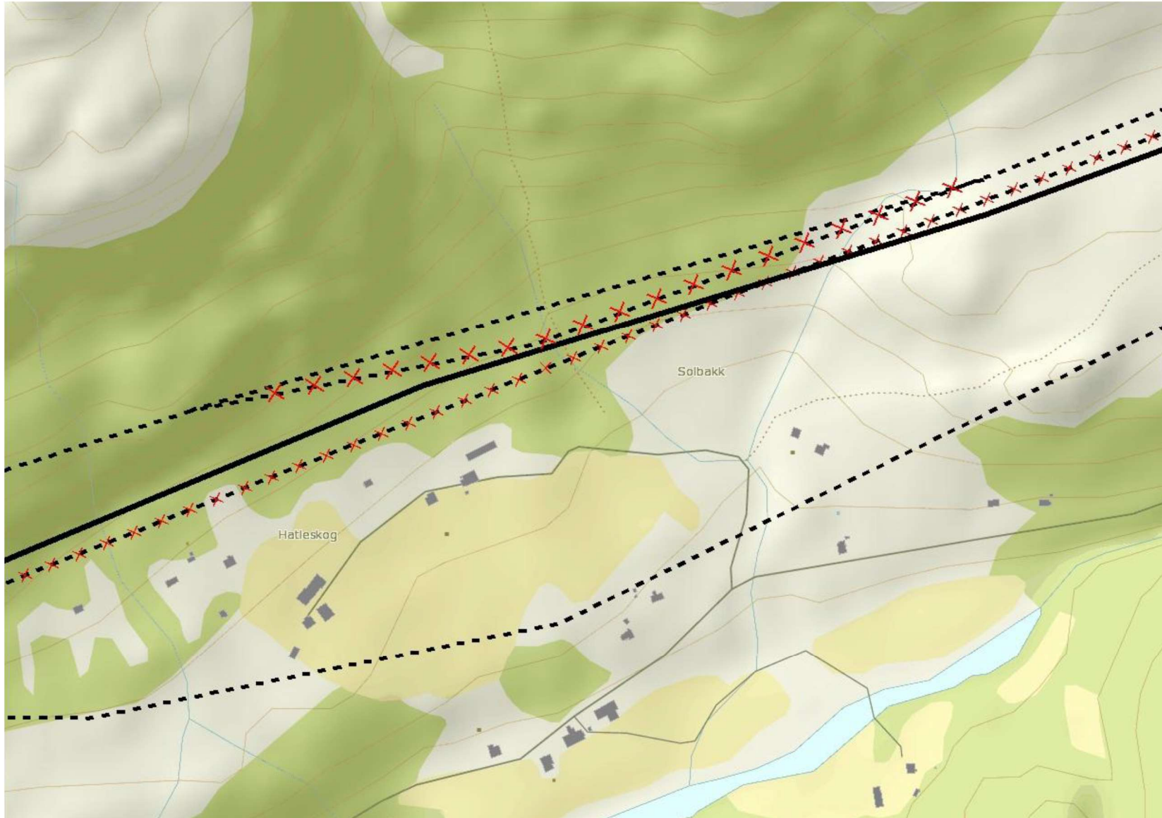
Omlegging av 132 kV kraftledning Lyse–Dalen ved Hatleskog (Konsesjonsøknad mai 2013)
