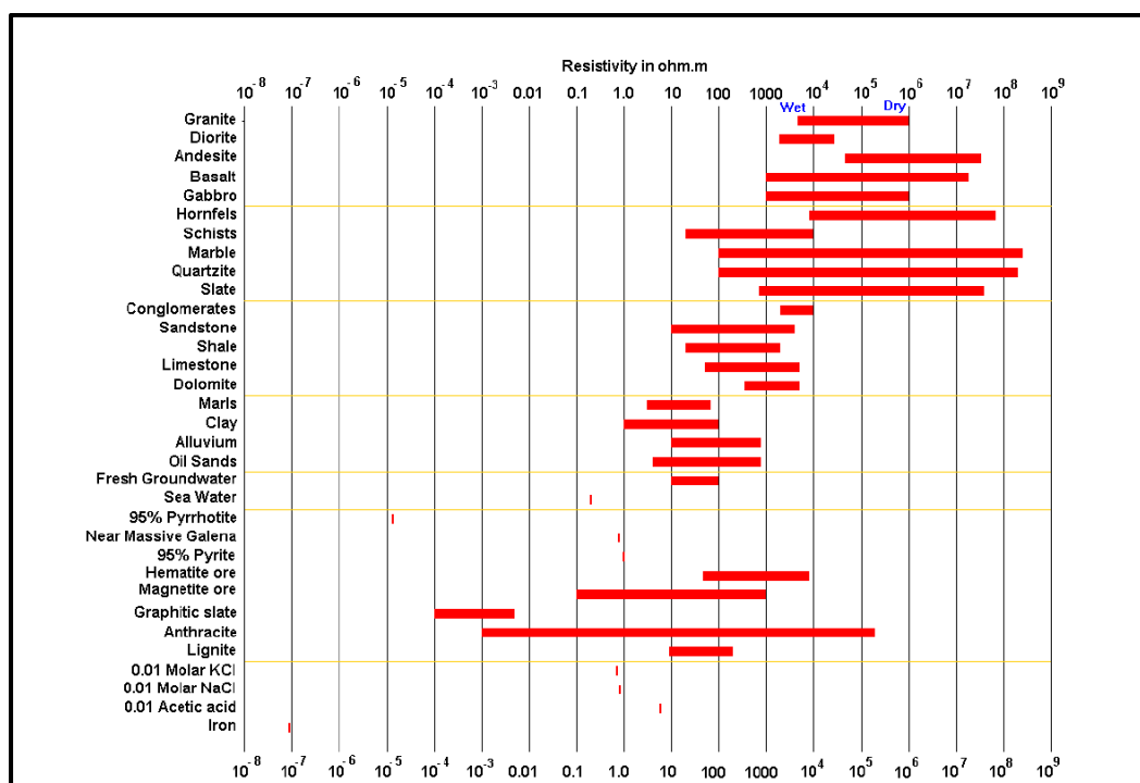
Figur 7: Resistivitet for ulike berg- og jordarter. (fra Loke M., 2004 Opplæring: 2-D og 3-D elektriske undersøkelser ).
