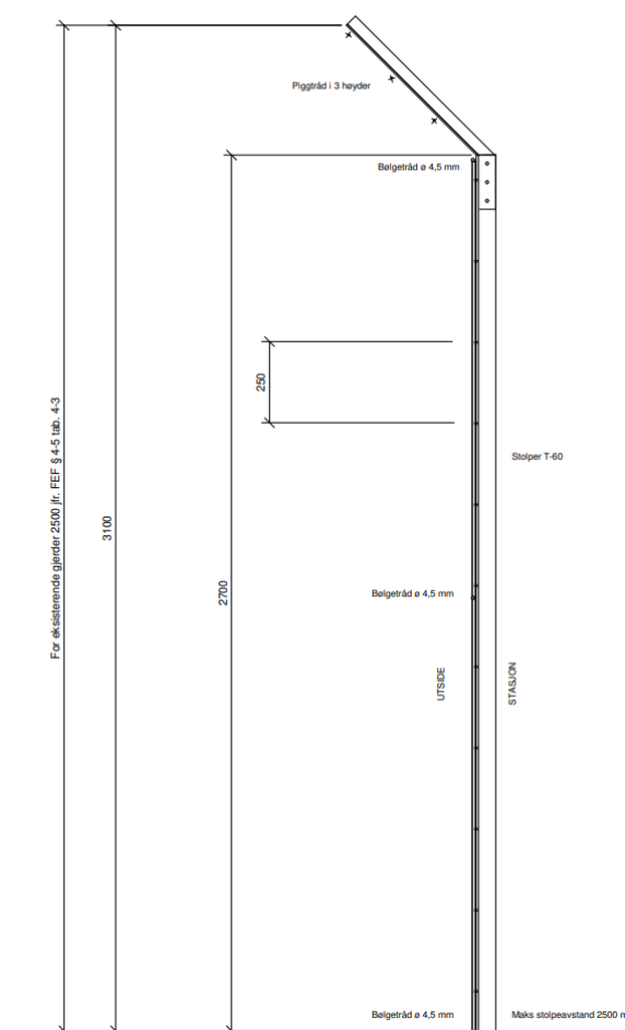
Figur 8. Standard stasjonsgjerde
