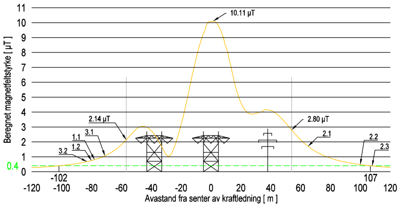
Figur 7 Magnetfelt for alternativ 1
