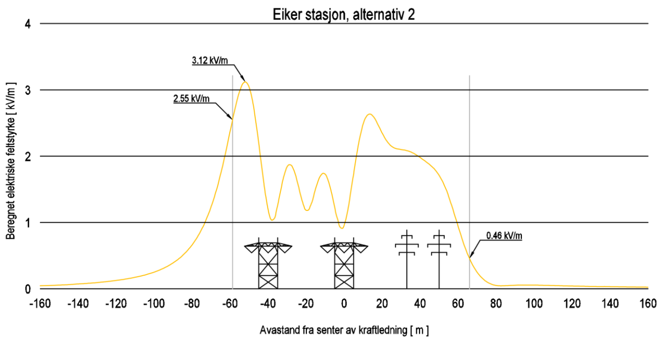
Figur 4 Elektrisk felt for alternativ 2
