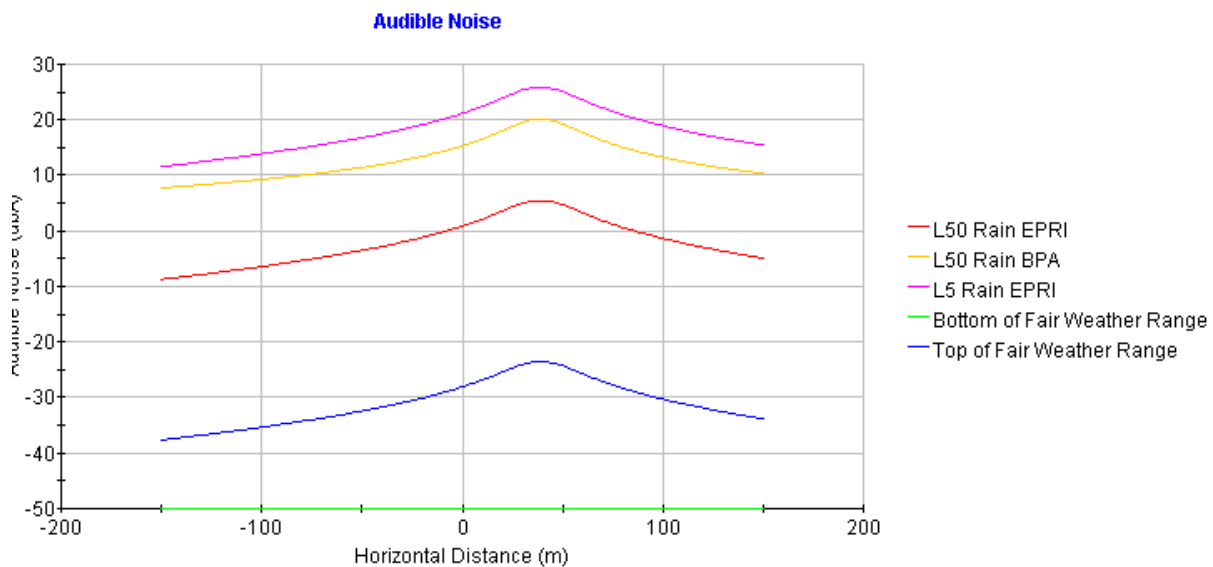
Figur 13 Hørbar støy for 145 kV dobbelt kurs
