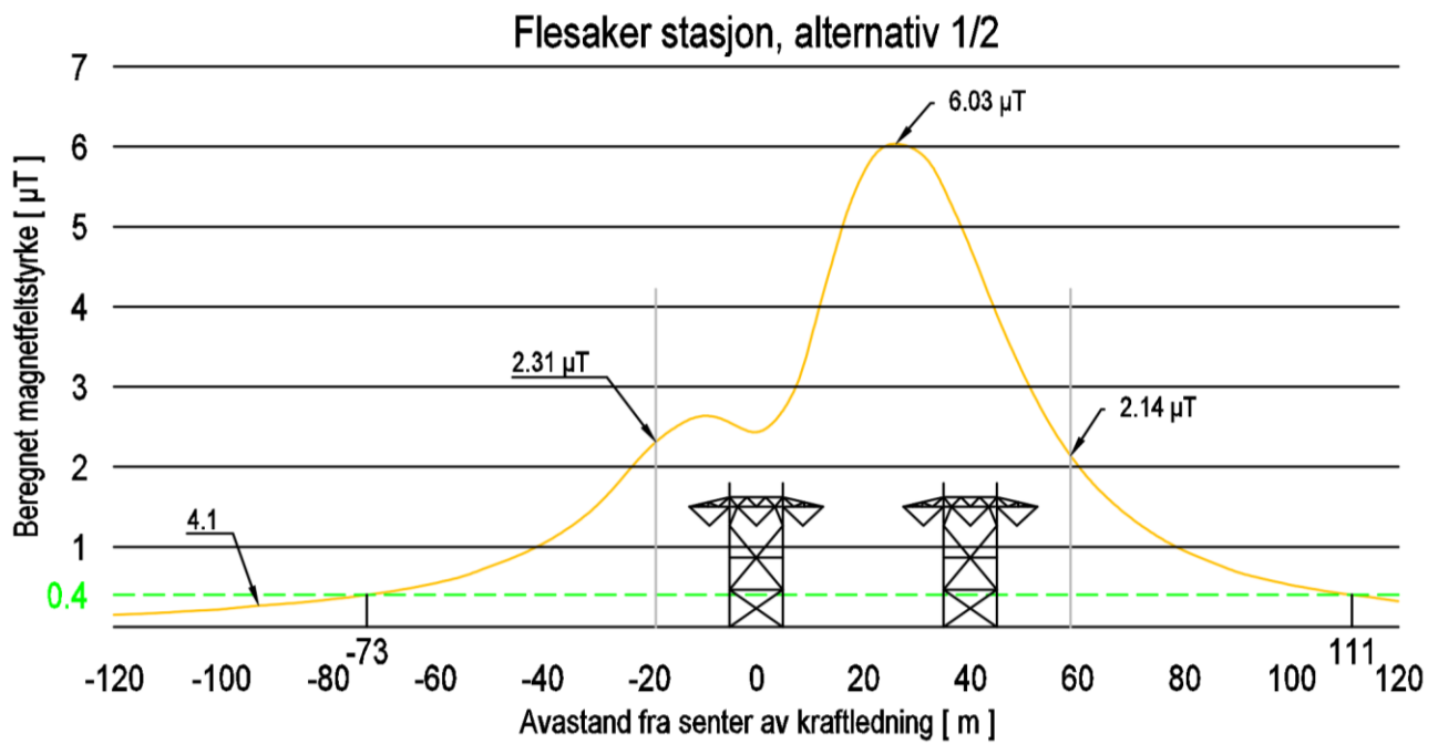
Figur 9 Magnetfelt rundt Flesaker stasjon, alternativ 1 og 2.
