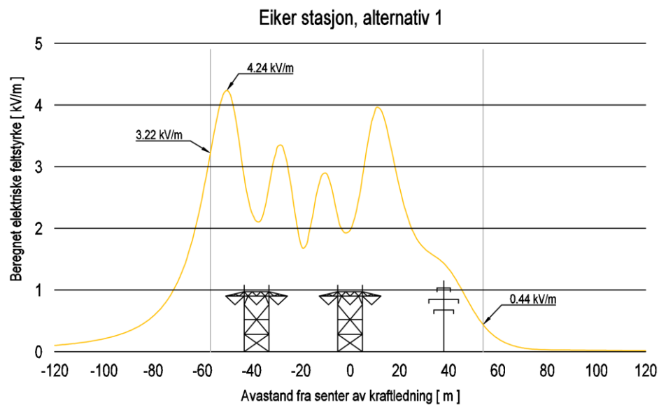
Figur 3 Elektrisk felt for alternativ 1
