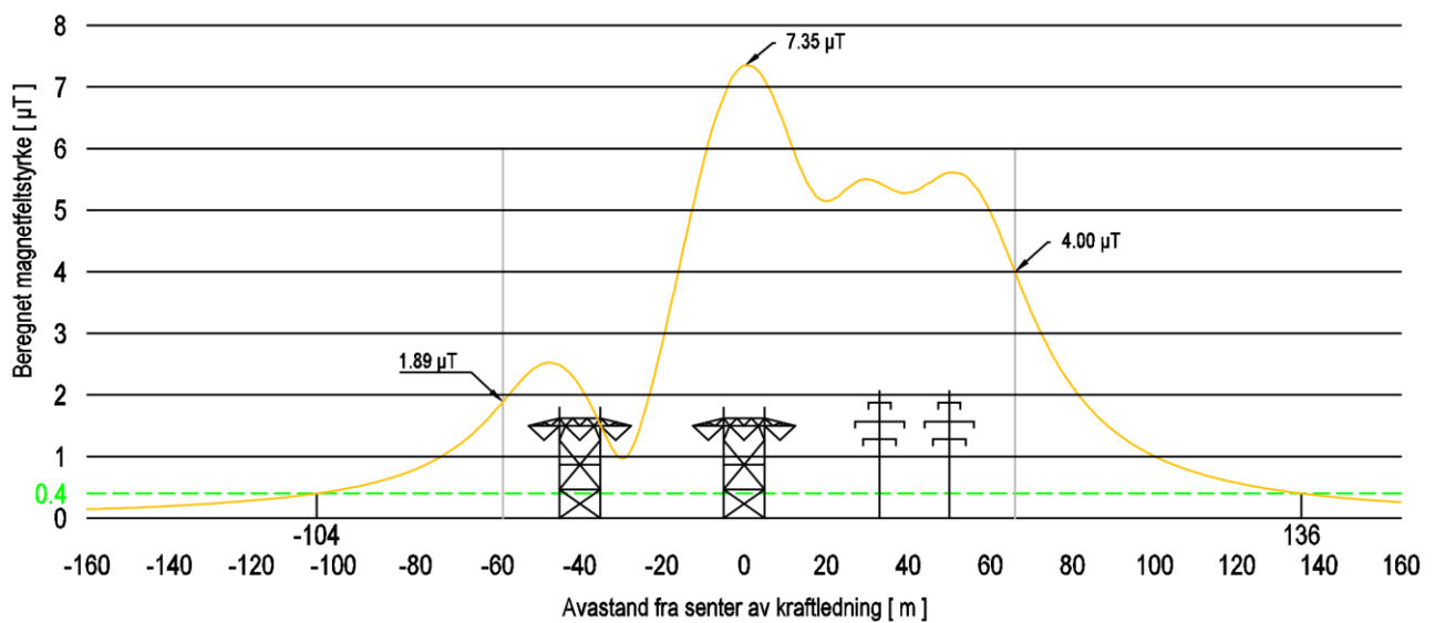
Figur 8 Magnetfelt for alternativ 2
