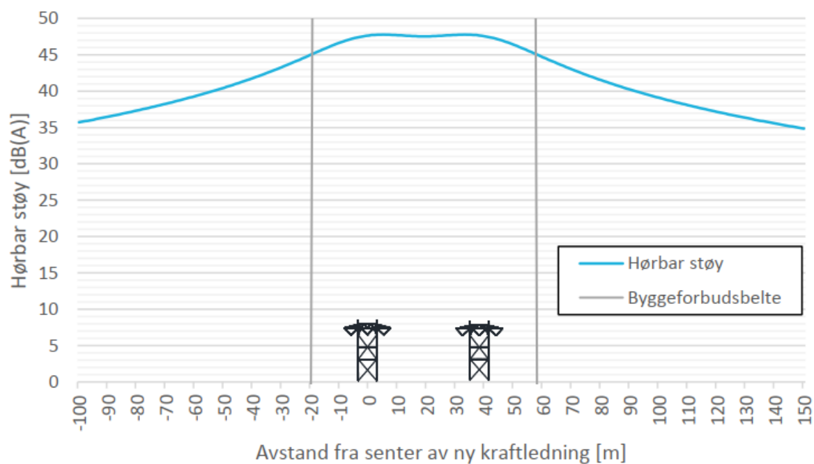
Figur 16 Hørbar støy for 2x420 kV tatt fra SDOK-39-50
