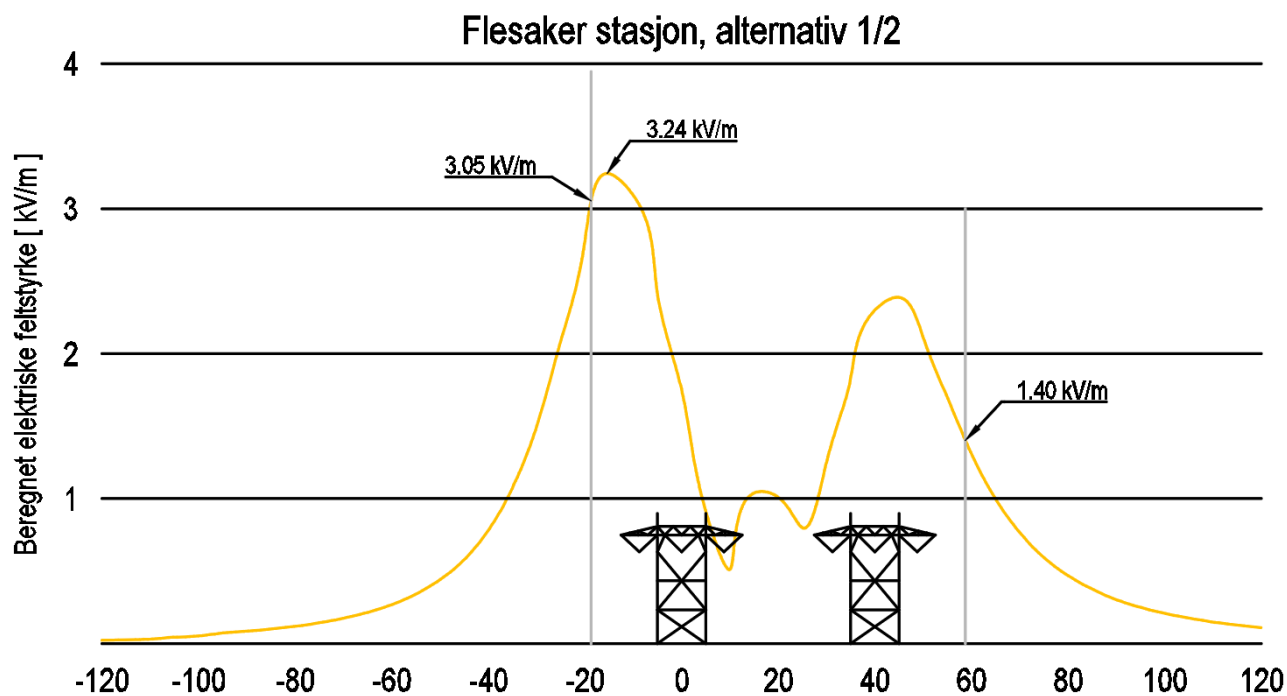
Figur 5 Elektrisk felt rundt Flesaker stasjon.
