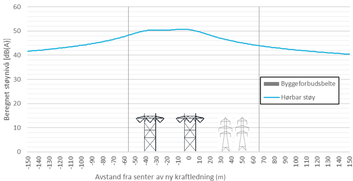
Figur 15 Hørbar støy for 2x420 kV og 4x145 kV
