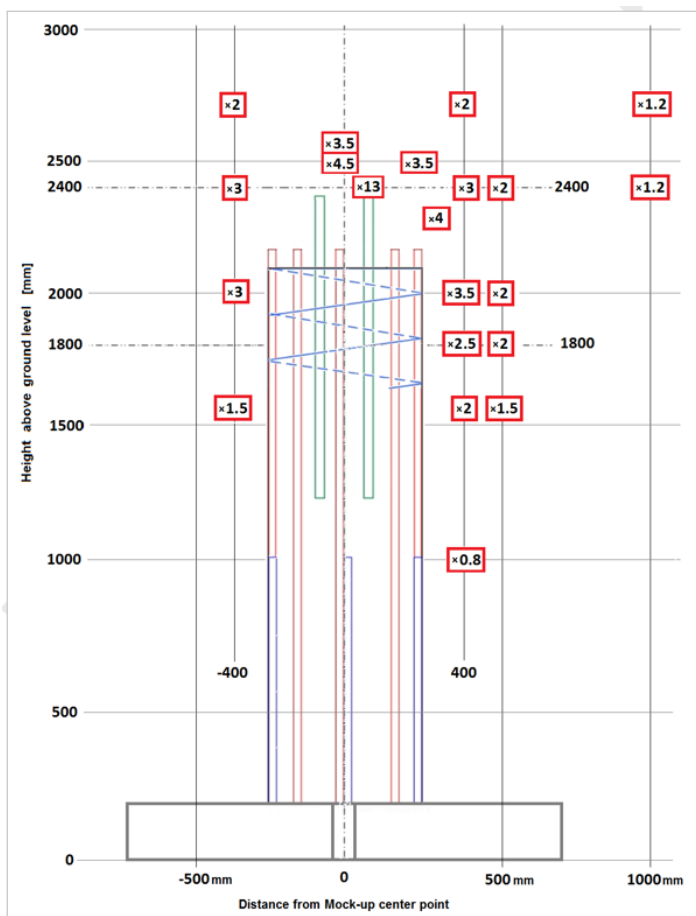
Figur 19: Beregnende forsterkningsfaktorer for E-felt ved mastefundament.
