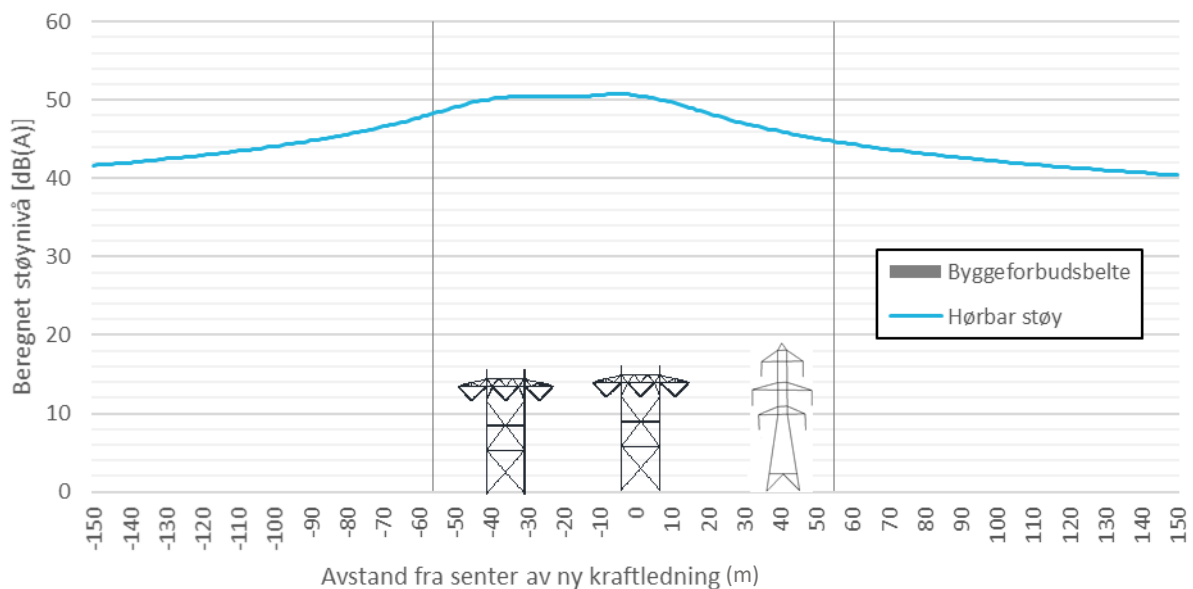
Figur 14 Hørbar støy for 2x420 kV og 2x145 kV
