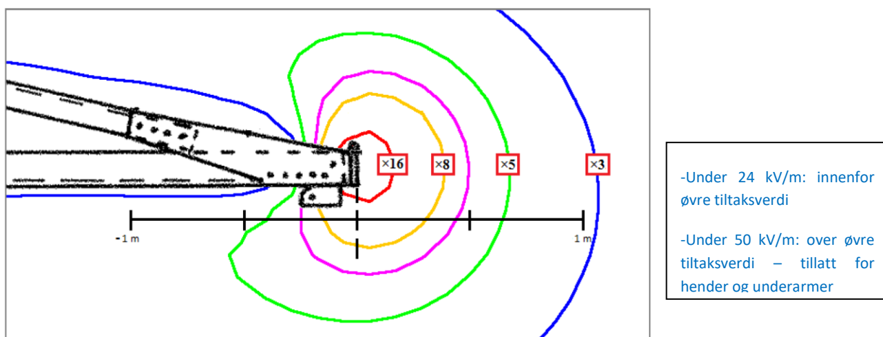
Figur 18: Beregnende forsterkningsfaktorer for E-felt ved traversspiss
