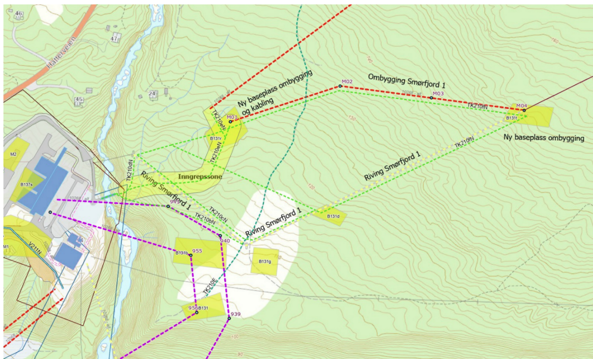
Figur 1. Arealbruk for omlegging av ledninger ved Skaidi stasjon. Det søkes om inngrepssone for kabling (kalt inngrepssone på kartet og vist med gult polygon på begge sider av kabeltraseen), kjørespor (TK210fN, TK210eN vist med grønne stiplede linjer) og baseplasser (B131r og B131t vist med gule polygoner). Resterende arealbruk som vises på kartet, er uendret. Kilde: Statnett, e-post av 22. april 2026.
