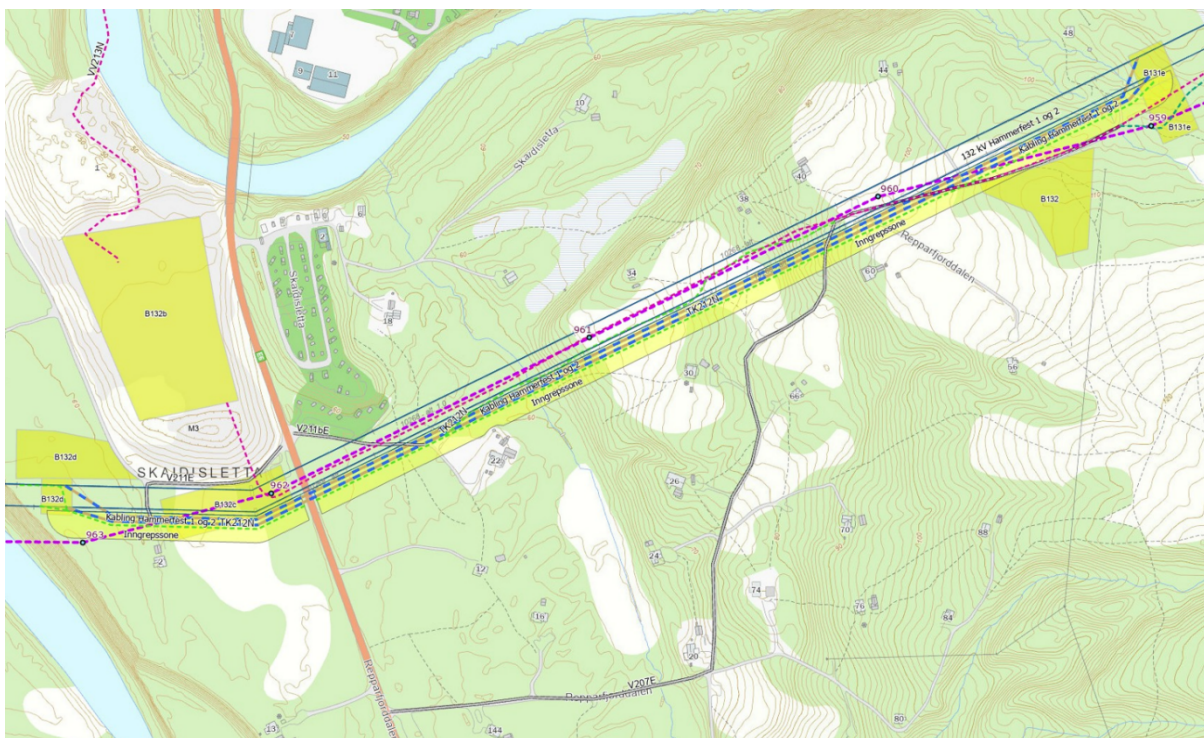
Figur 2. Arealbruk for kabling av 132 kV Hammerfest 1 og 2. Det søkes om inngrepssone for kabling for midlertidig lagring av masser og midlertidig kjørespor (TK212N). Kilde: Statnett, e-post av 22. april 2026.
