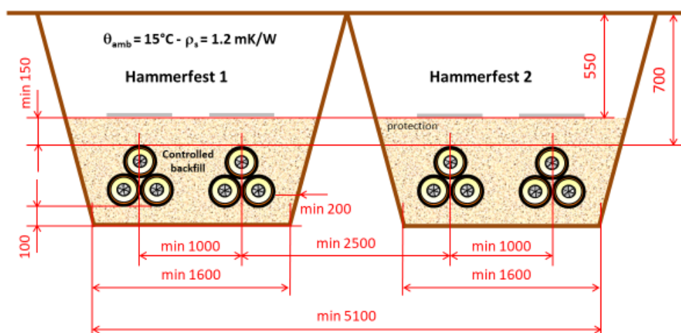
Figur 6. Snitt som viser kabelgrøft for kabling av 132 kV Hammerfest 1 og 2 som tilhører Lucerna.
