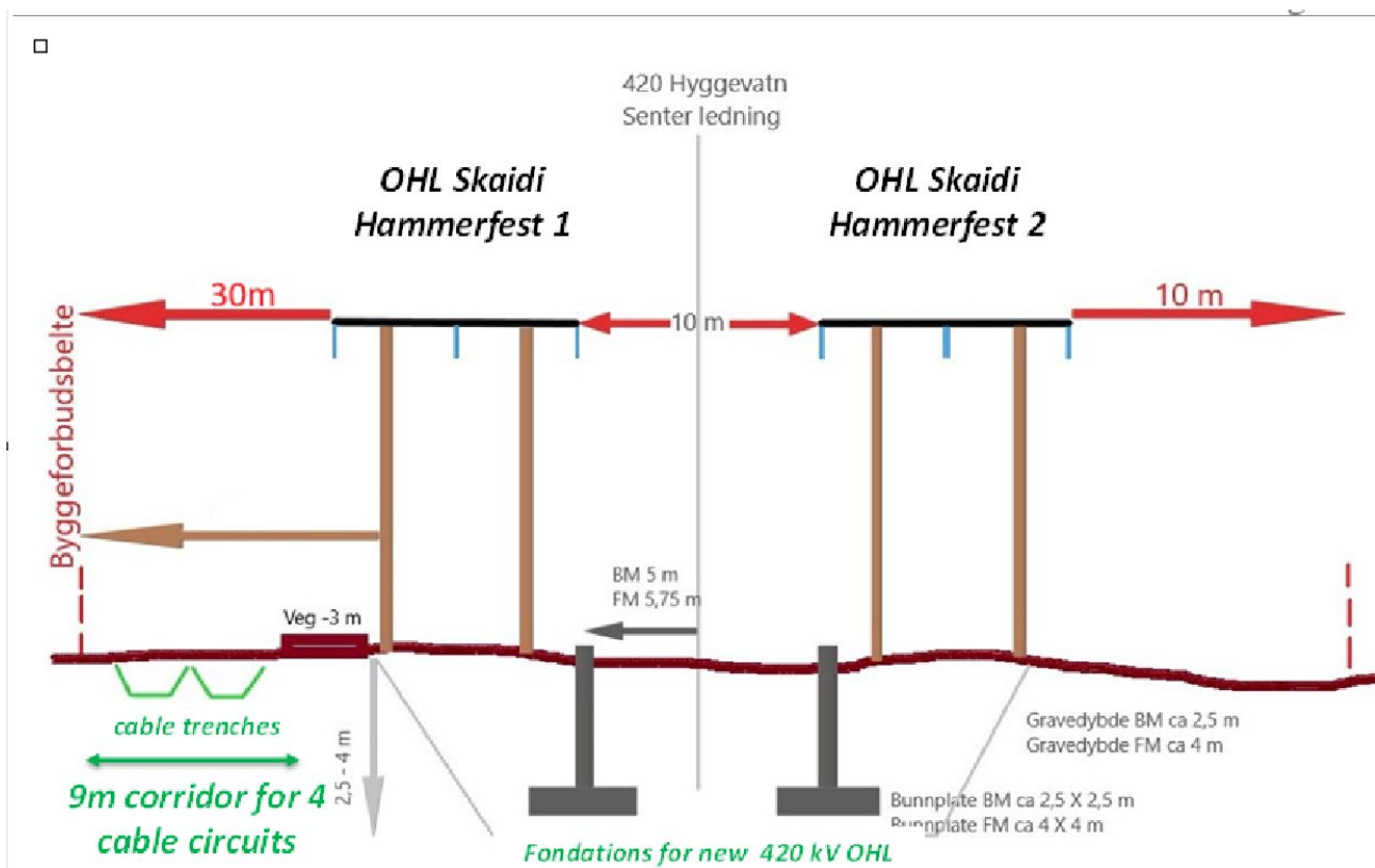
Figur 2 Prinsippskisse kabelgrøft og inngressone
