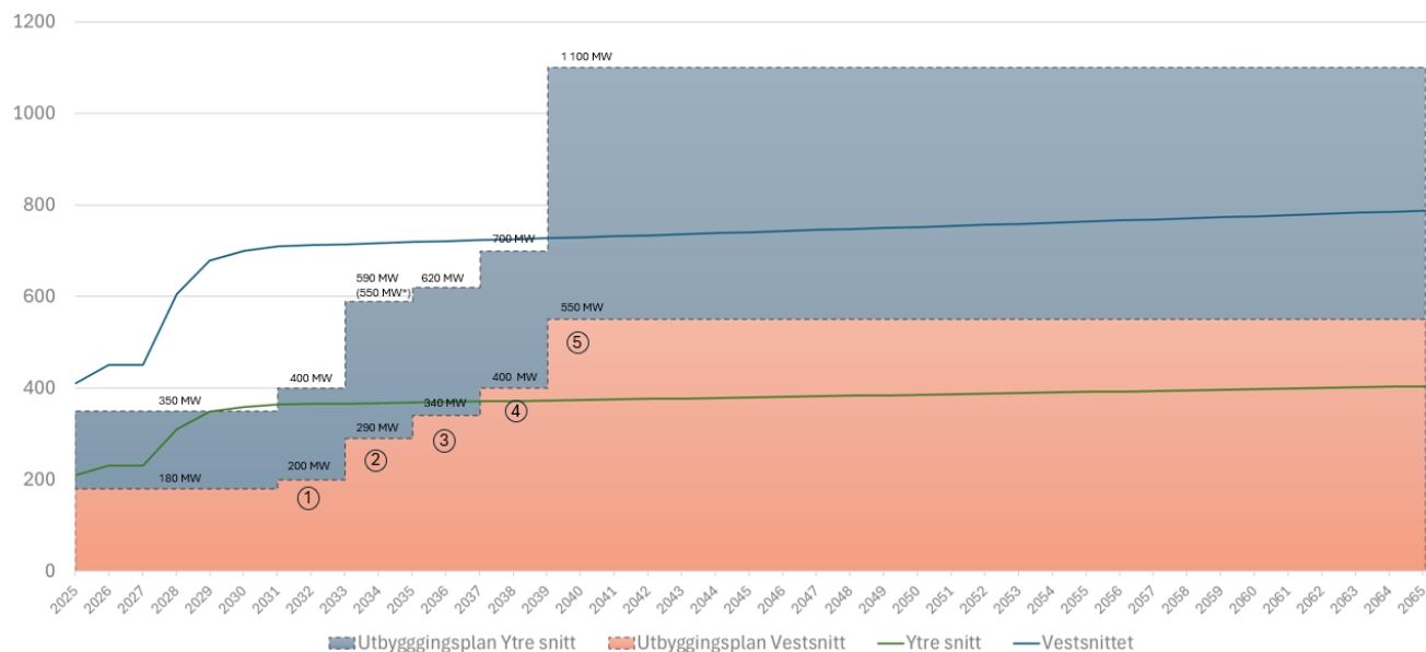
Figur 12: Overføringskapasitet og utbyggingstakt vs. lastprognosen i middelscenarioet
