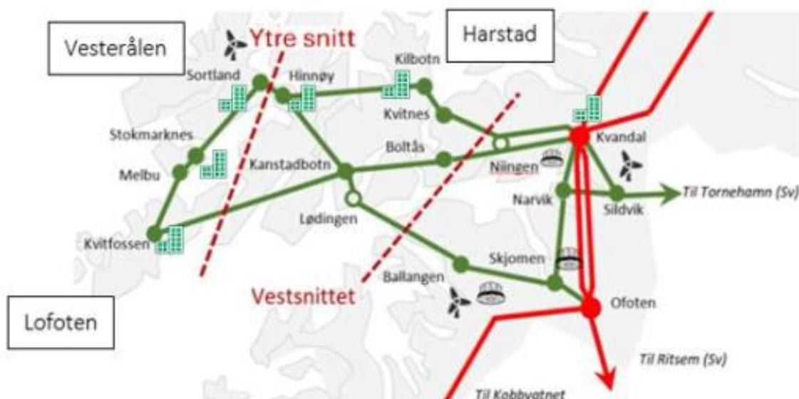
Figur 1: Dagens nettløsning for Lofoten og Vesterålen
