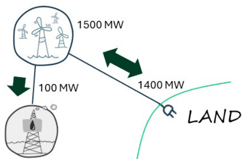
Figur 14: Illustrasjon av samlokalisering med utgangspunkt i havvind .
