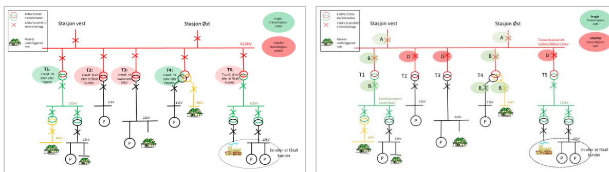
Figur 1 - Klassifisering av transformatorer og bryterfelt
