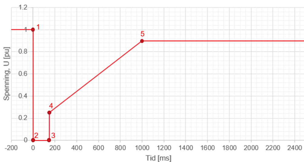
FIGUR 12-12: KRAV TIL FAULT RIDE THROUGH FOR TYPE D TILKNYTTET SPENNINGSNIVÅ \geq 110 \text{ kV} . PRODUKSJONSENHETEN SKAL VÆRE TRANSIENT STABIL OG BEHOLDE SYNKRONISME FOR ALLE FEILFORLØP SOM GIR ET SPENNINGSFORLØP I TILKNYTNINGSPUNKTET SOM LIGGER OVER KURVEN.
