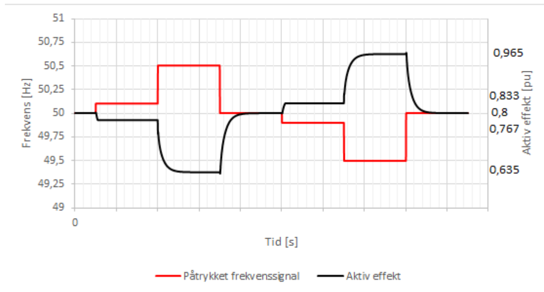
FIGUR 16-4: ILLUSTRASJON AV PRØVE FOR AKTIV EFFEKTPRESPONS (SORT) VED PÅTRYKKET FREKVENSSTEG (RØD).
