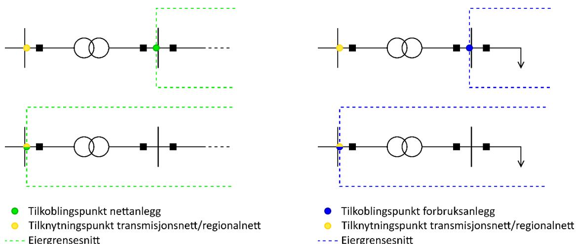
FIGUR 10-1 TILKOBLINGSPUNKT KAN VÆRE PÅ LAVSPENTSIDE AV TRANSFORMATOR TILKNYTTET REGIONAL- ELLER TRANSMISJONSNETT, VED EIERGRENSESNIITT. MEN TILKNYTNINGSPUNKTET VIL ALLTID VÆRE PÅ HØYSPENTSIDE AV TRANSFORMATOREN.
