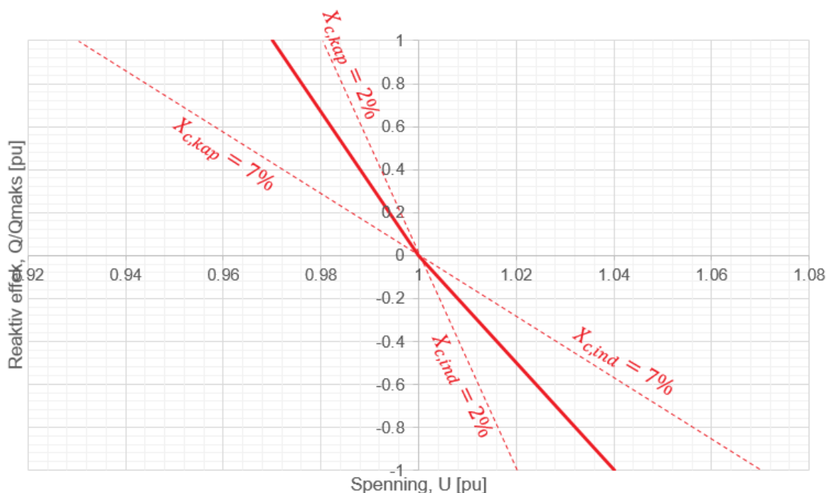
FIGUR 18-5: REAKTIV EFFEKT SOM FUNKSJON AV SPENNING I SPENNINGSREGULERINGSMODUS FOR HVDC-SYSTEMET.
