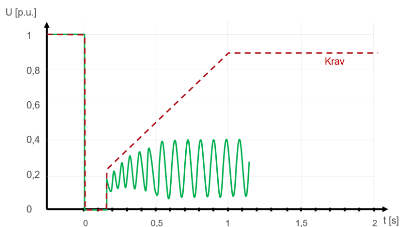
FIGUR 13-3: TYPISK TIDSFØRSLØP FOR SPENNING I TILKNYTNINGSPUNKT NÅR SYNKRONISME MOT NETTET TAPES VED FEILKLARERINGSSTID > CCT, NÅR SPENNINGEN ETTER FEIL LIGGER UNDER KRAVKURVEN.
