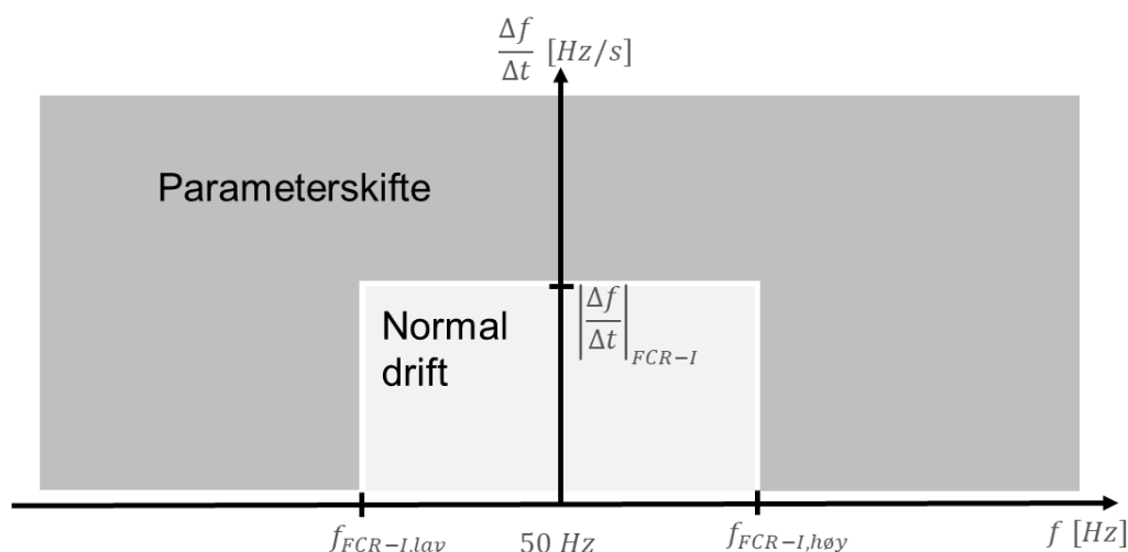
FIGUR 12-5: ILLUSTRASJON AV AUTOMATISK OG UFORSINKET AKTIVERING AV FSM VED KITERIER FOR FCR-I.
