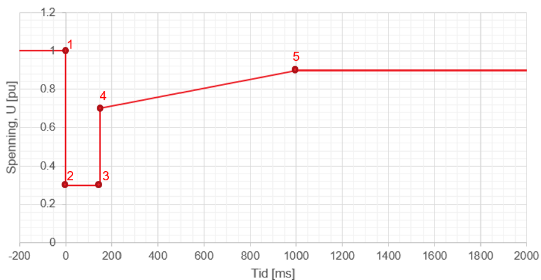
FIGUR 12-11: KRAV TIL FAULT RIDE THROUGH FOR TYPE A, B OG C, SAMT TYPE D TILKNYTTET SPENNINGSNIVÅ < 110 \text{ kV} . PRODUKSJONSENHETEN SKAL VÆRE TRANSIENT STABIL OG BEHOLDE SYNKRONISME FOR ALLE FEILFORLØP SOM GIR EN SPENNING I TILKNYTNINGSPUNKTET SOM LIGGER OVER KURVEN.
