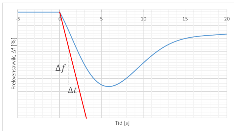
FIGUR 14-2: ILLUSTRASJON AV KRAV TIL FREKVENSENDRINGSKRAV. DERSOM FREKVENSFORLØPET ER OVER DEN RØDE LINJEN, SOM FALLER MED EN FREKVENSENDRINGSKRAV PÅ \frac{\Delta f}{\Delta t} = 1,5 \text{ Hz/s} , SKAL PRODUKSJONSENHETEN OPERERE NORMALT.
