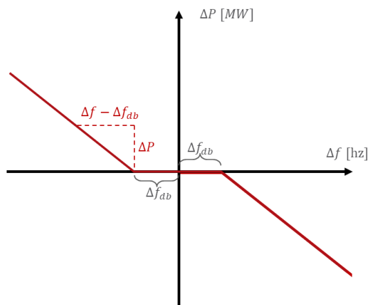
FIGUR 12-4: REGULATORRESPONS SOM FUNKSJON AV FREKVENSI I FREKVENSSREGULERINGSMODUS FOR SYNKRONE PRODUKSJONSENHETER.
