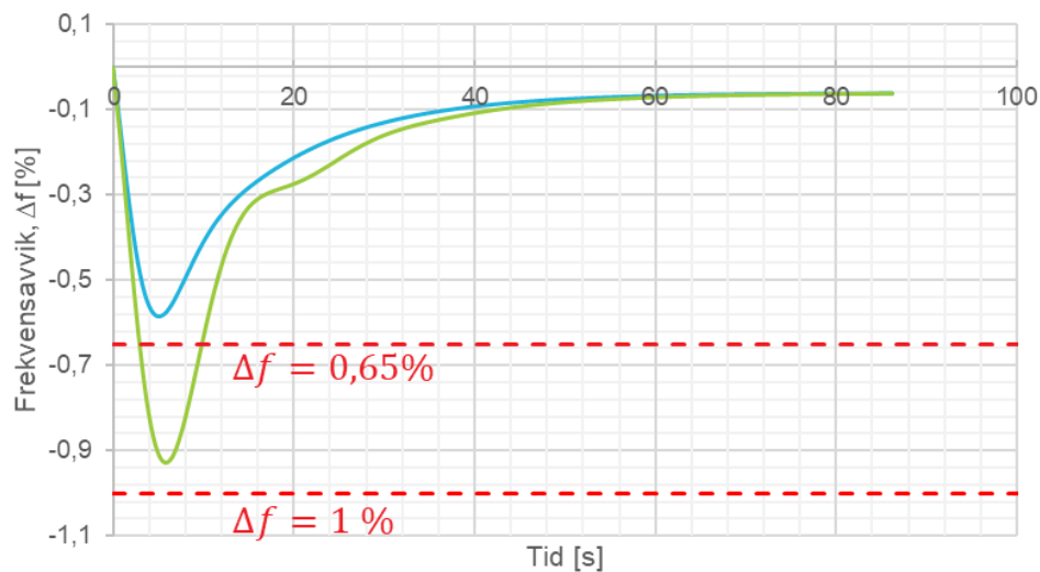
FIGUR 13-10: FREKVENSPRESPONS I TIDSPLANET VED 1 % LASTPÅSLAG REFERERT P_{maks} , VED P_{sett} = 85 \% \cdot P_{maks} OG 2 % STATIKK. DE RØDE STIPLEDE LINJENE REPRERENTERER KRAVENE TIL MAKSIMALT TRANSIENT FREKVENSAVVIK. GRØNN (TYPE B OG C) OG BLÅ KURVER (TYPE D) ER EKSEMPLER PÅ FREKVENSFØRLØP ETTER ET LASTSPRANG PÅ EGET OHMSK NETT.
