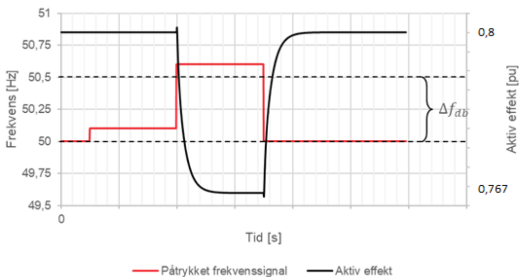
FIGUR 13-25: ILLUSTRASJON AV PRØVE FOR AKTIV EFFEKTRESPONS (SORT) VED PÅTRYKKET FREKVENSSTEG(RØD) MED AKTIVE DØDBÅND (SORT STIPLET LINJE).
