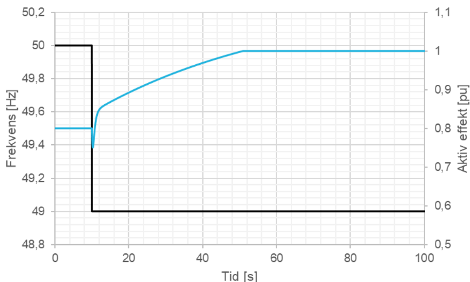
FIGUR 13-28: ILLUSTRASJON AV PRØVE AV AKTIV EFFEKTTRESPONS (BLÅ) VED DETEKSJON AV SEPARATDRIFT VED HØY FREKVENSENDRINGSFASTIGHET ( \Delta f / \Delta t , ROCOF) VED PÅTRYKKET FREKVENSRAMPE (SORT).
