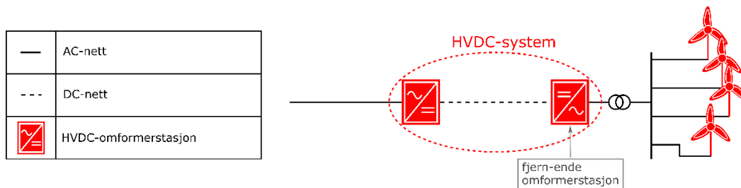
FIGUR 17-2: ILLUSTRASJON AV HVDC-SYSTEM MED FJERN-ENDE HVDC-OMFORMER
