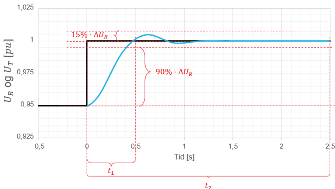
FIGUR 13-32: ILLUSTRASJON AV PRØVER FOR DOKUMENTASJON AV KRAV TIL UTREGULERINGSTID AV SPENNINGSREFERANSESTEG I POSITIV RETNING FOR MAGNETISERINGSUTSTYR MED ÅPNE GENERATORKLEMMER FOR SYNKRONE PRODUKSJONSENHETER.
