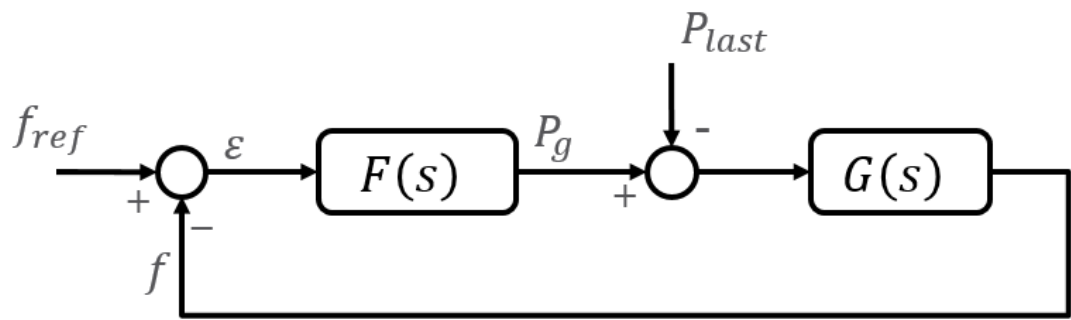
FIGUR 13-12: LUKKET SLØYFE
