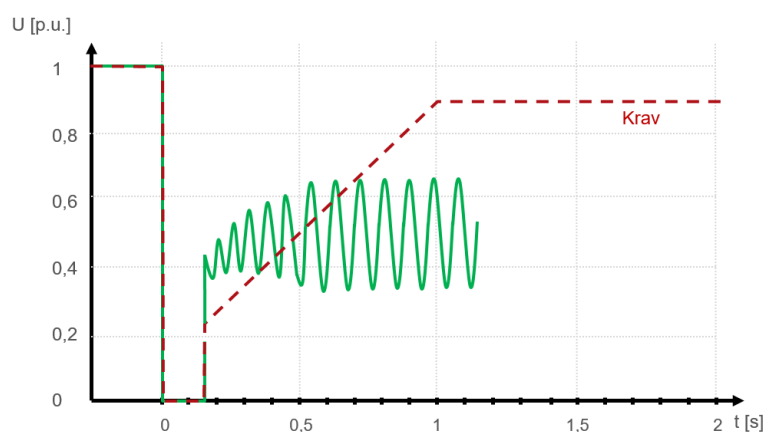
FIGUR 13-2: TYPISK TIDSFØRSLØP FOR SPENNING I TILKNYTNINGSPUNKT NÅR SYNKRONISME MOT NETTET TAPES VED FEILKLARERINGSSTID > CCT, SELV OM SPENNINGEN LIGGER OVER KRAV-SPENNINGSPROFILEN.
