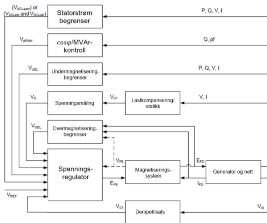
FIGUR 13-14: PRINSIPIELL VIRKEMÅTE TIL SPENNINGSREGULATOREN FOR EN SYNKRON PRODUKSJONSENHET [11]. NB; MERK AT BLOKKDIAGRAMMET KUN VISER SPENNINGSINNGANG TIL DEMPETILSATS. DEMPETILSATS SKAL OGSÅ BENYTTET IHT. KRAV I KAPITTEL 12.5.6.
