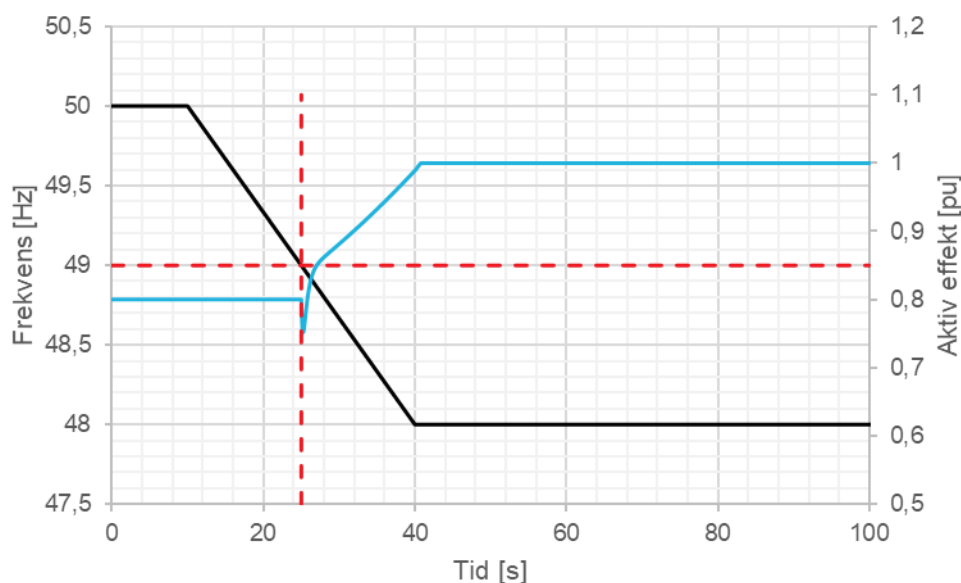
FIGUR 13-27: ILLUSTRASJON AV PRØVE AV AKTIV EFFEKTRESPONS (BLÅ) VED DETEKSJON AV SEPARATERDRIFT VED FREKVENSTERSKEL VED PÅTRYKKET FREKVENSRAMPE (SORT). BLÅ KURVE VISER ENDRING I PARAMETERSETT VED FREKVENNS < 49 Hz.
