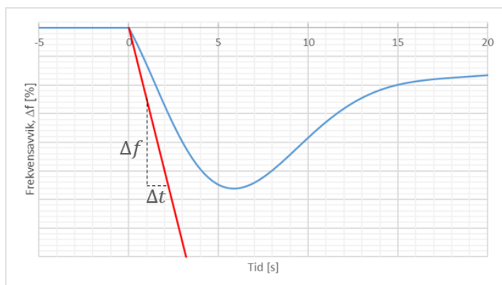
FIGUR 12-3: ILLUSTRASJON AV KRAV TIL FREKVENSENDERINGSFASTIGHET. DERSOM FREKVENSFORLØPET ER OVER DEN RØDE LINJEN, SOM FALLER MED EN FREKVENSENDERINGSFASTIGHET PÅ \frac{\Delta f}{\Delta t} = 1,5 \text{ Hz/s} , SKAL PRODUKSJONSENHETEN OPERERE NORMALT.
