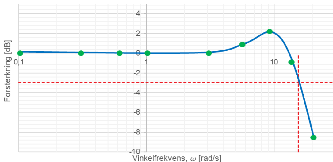
FIGUR 13-35: ILLUSTRASJON AV MAGNETISERINGSSYSTEMETS LUKKET SLØYFE-FORSTERKNING (BLÅ), MED BÅNDBREDDE ILLUSTRERT (RØDSTIPLET). GRØNNE SIRKLER ILLUSTRERER DE TESTEDE PÅTRYKTE FREKVENSENE SOM ER TESTET.
