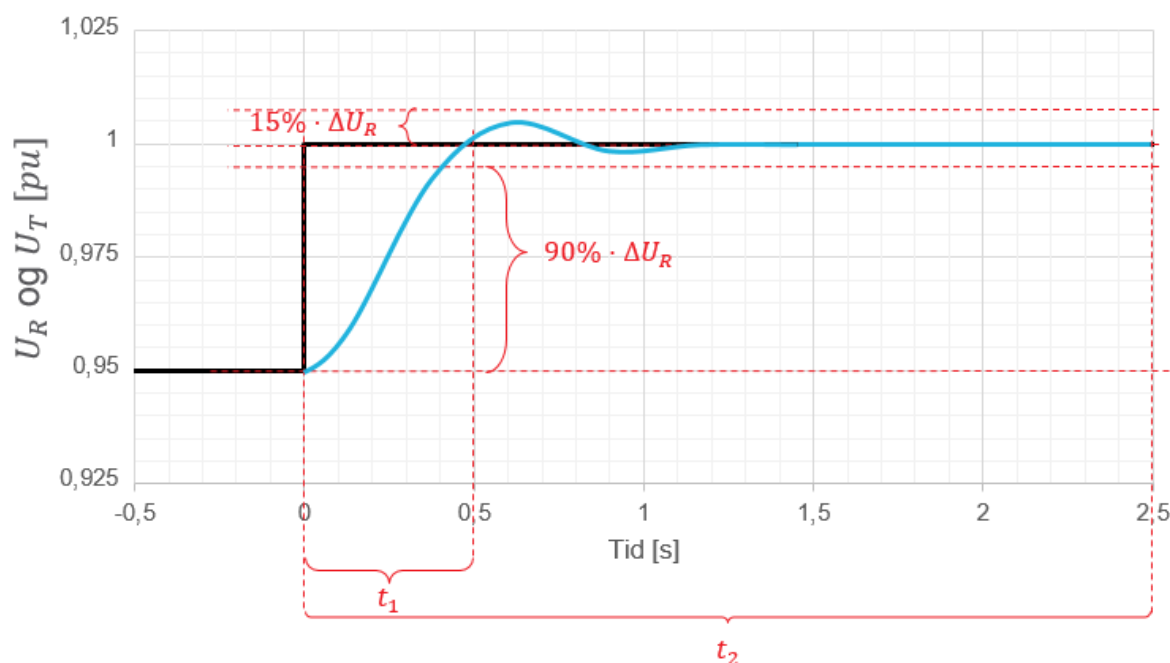
FIGUR 13-15: ILLUSTRASJON AV KRAV TIL UTREGULERINGSTID AV SPENNINGSREFERANSESTEG I POSITIV RETNING FOR MAGNETISERINGSUTSTYR I LUKKET SLØYFE MED ÅPEN EFFEKTBRYTER FOR SYNKRONE PRODUKSJONSENHETER.
