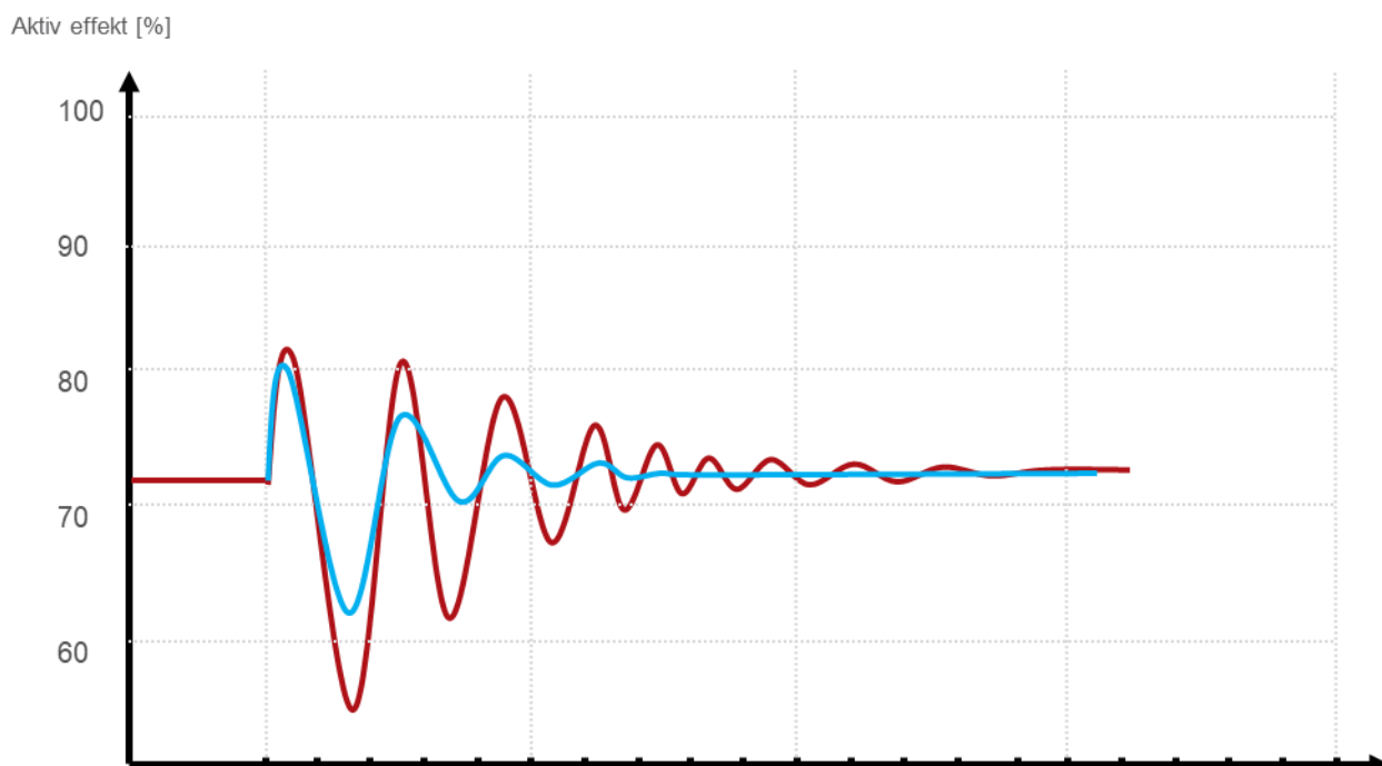
FIGUR 13-34: ILLUSTRASJON AV DEMPETILSATSENS EFFEKT PÅ EFFEKTPENDLINGER ETTER EN PÅTRYKKET SPENNINGSIMPULS. BLÅ VISER AKTIV EFFEKTRESPONS MED AKTIV DEMPETILSAT, OG RØD VISER AKTIV EFFEKTRESPONS UTEN DEMPETILSAT.
