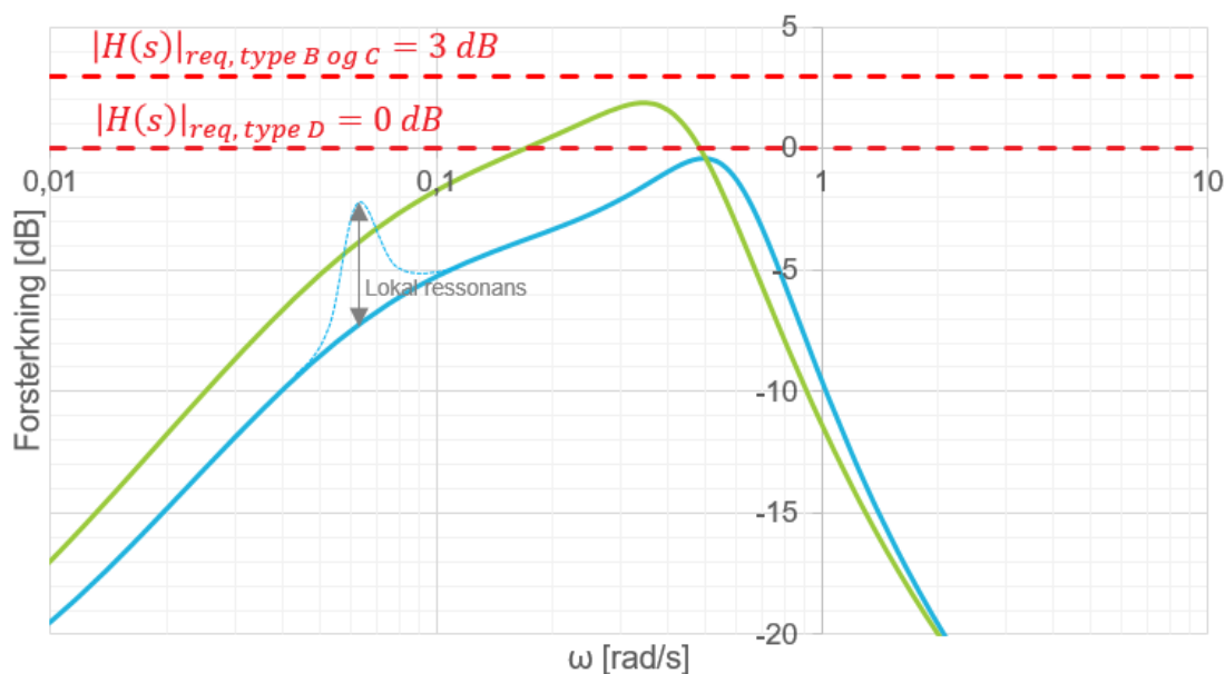
FIGUR 13-11: FREKVENSPRESPONS ILLUSTRERT I FREKVENSPLANET VED 1 % LASTPÅSLAG REFERERT P_{maks} , VED P_{sett} = 0,85 \cdot P_{maks} OG 2 % STATIKK. DE RØDE STIPLEDE LINJENE REPRERENTERER KRAVENE TIL MAKSIMALT TRANSIENT FREKVENSAVVIK. GRØNN (TYPE B OG C) OG BLÅ KURVER (TYPE D) ER EKSEMPLER PÅ FREKVENSFØRLØP ETTER ET LASTSPRANG PÅ EGET OHMSK NETT.
