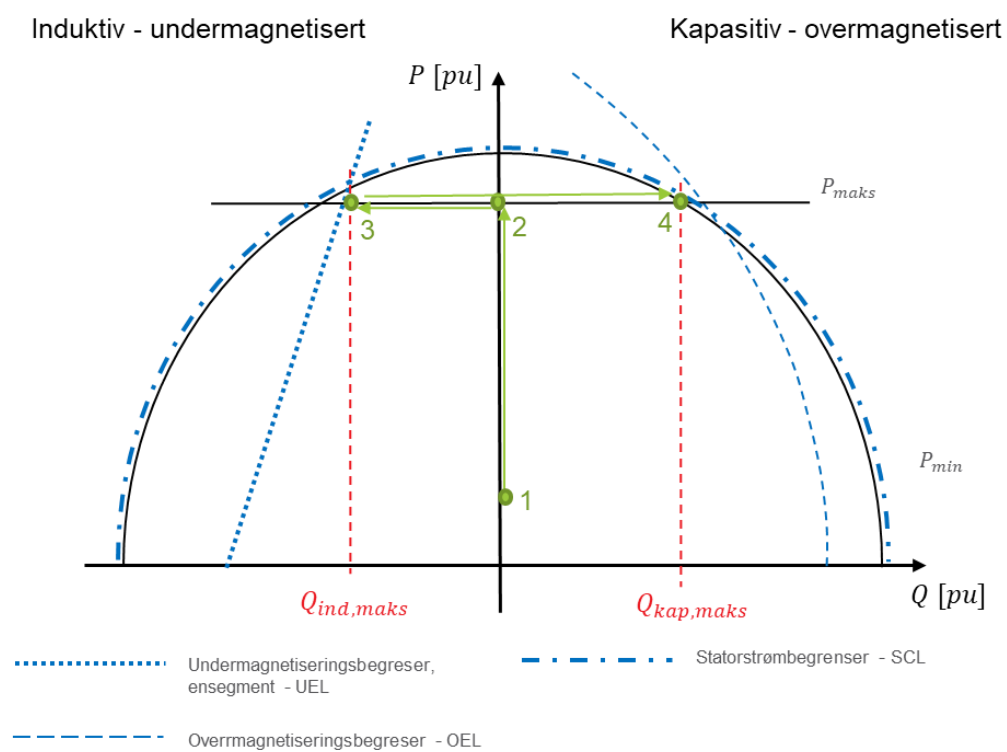
FIGUR 13-36: ILLUSTRASJON AV METODE FOR GJENNOMFØRING AV TEST AV REAKTIV YTELSE FOR SYNKRONE PRODUKSJONSENHETER. GRØNNE PUNKTER HENVISER TIL PUNKTLISTE OVER.
