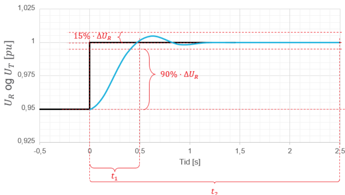
FIGUR 12-8: ILLUSTRASJON AV KRAV TIL UTREGULERINGSTID AV SPENNINGSREFERANSESTEG I POSITIV RETNING FOR MAGNETISERINGSUTSTYR I LUKKET SLØYFE MED ÅPEN EFFEKTBYTER FOR SYNKRONE PRODUKSJONSENHETER.
