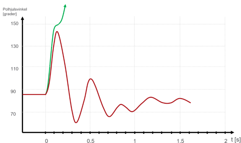
FIGUR 13-4: TYPISK TIDSFØRSLØP FOR ROTORVINKEL I TILKNYTNINGSPUNKT NÅR SYNKRONISME MOT NETTET BEHOLDNES (RØD) OG TAPES (GRØNN).
