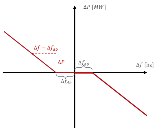
FIGUR 18-2: REGULATORRESPONS SOM FUNKSJON AV FREKVEN I FREKVENSRGULERINGSMODUS FOR HVDC-SYSTEMER
