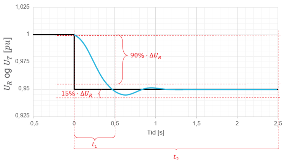
FIGUR 12-9: ILLUSTRASJON AV KRAV TIL UTREGULERINGSTID AV SPENNINGSREFERANSESTEG I NEGATIV RETNING FOR MAGNETISERINGSUTSTYR I LUKKET SLØYFE MED ÅPEN EFFEKTBYTER FOR SYNKRONE PRODUKSJONSENHETER.
