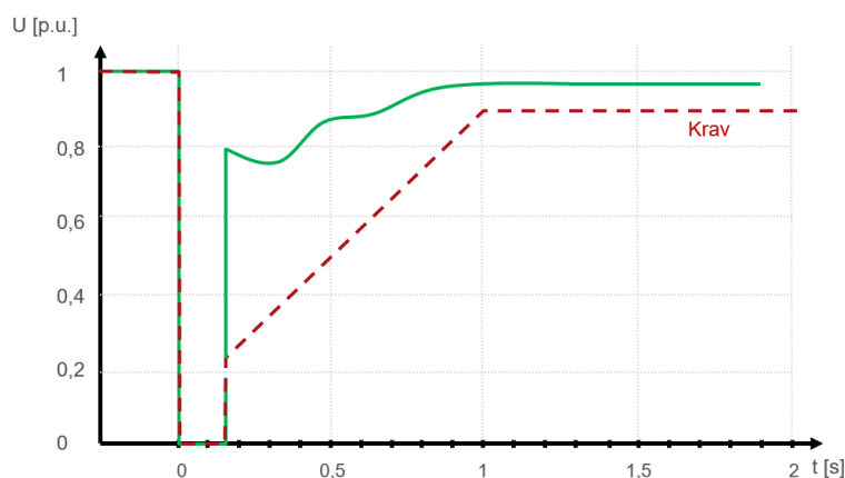
FIGUR 13-1: TYPISK TIDSFØRSLØP FOR SPENNING I TILKNYTNINGSPUNKT NÅR SYNKRONISME MOT NETTET BEHOLDNES.
