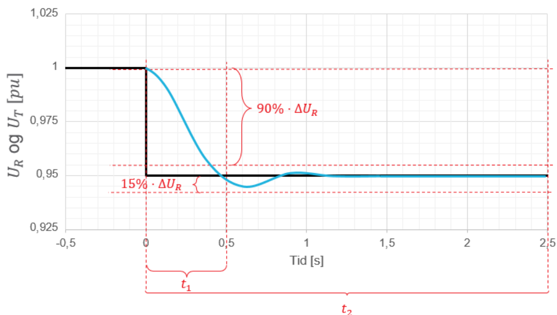
FIGUR 13-33: ILLUSTRASJON AV PRØVER FOR DOKUMENTASJON AV KRAV TIL UTREGULERINGSTID AV SPENNINGSREFERANSESTEG I NEGATIV RETNING FOR MAGNETISERINGSUTSTYR MED ÅPNE GENERATORKLEMMER FOR SYNKRONE PRODUKSJONSENHETER.
