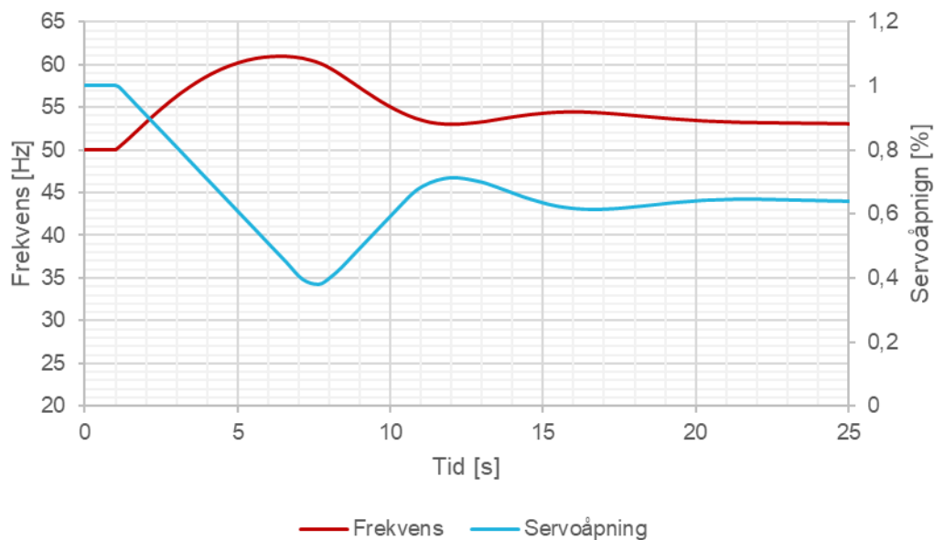
FIGUR 13-13: ILLUSTRASJON AV SIMULERING AV ET STORT LASTSPRANG HVOR ULINEARITETER ER DOMINERENDE, HER SYNLI VED VENTILMETNING I OLJETRYKKANLEGG, SOM GIR KONSTANT ENDRINGSHASTIGHET PÅ SERVOÅPNING.
