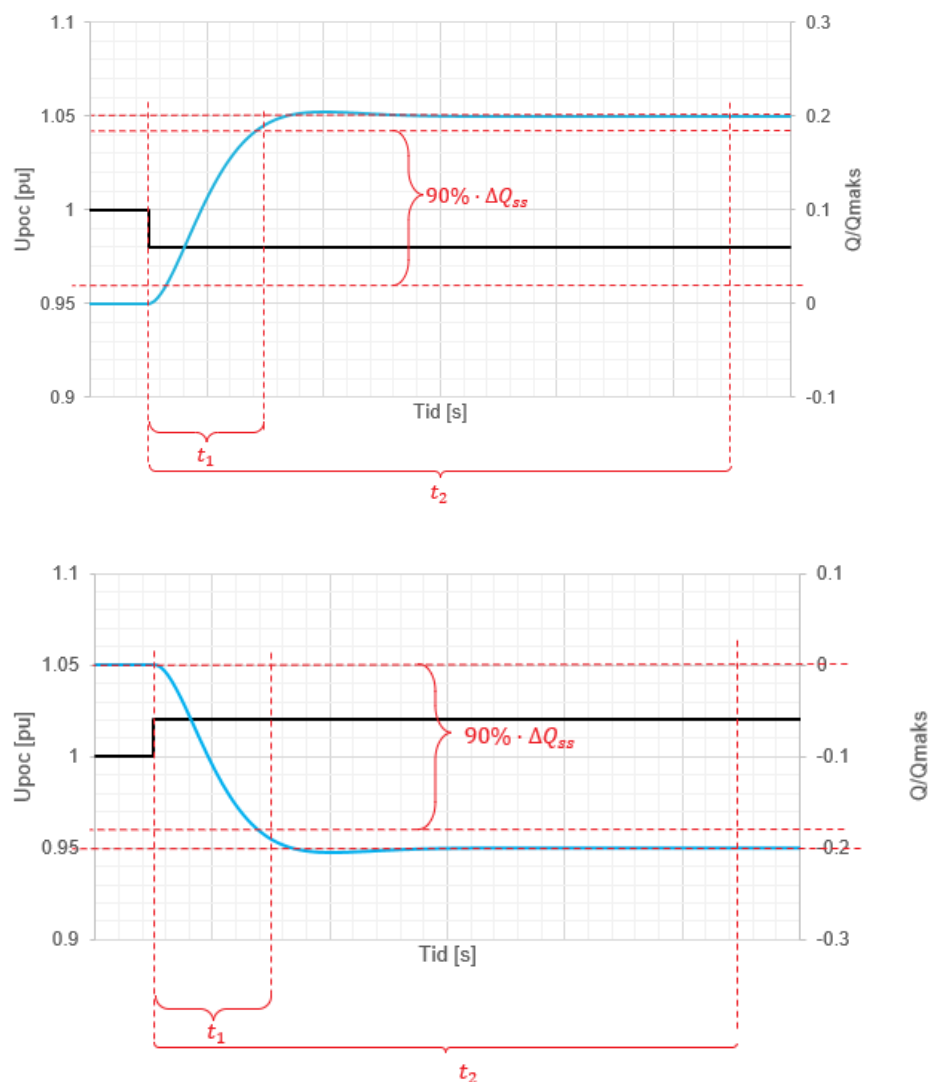
FIGUR 18-6: REAKTIV EFFEKTPRESPONS VED STEGVIS ENDRING I SPENNING PÅ HHV -/+ 2\% . KRAV ER MARKERT I RØDSTIPLEDE LINJER
