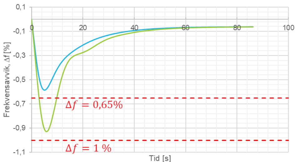
FIGUR 12-6: FREKVENSPRESPONS I TIDSPLANET VED 1 % LASTPÅSLAG REFERERT P_{maks} , VED P_{sett} = 85 \% \cdot P_{maks} OG 2 % STATIKK. DE RØDE STIPLEDE LINJENE REPRERENTERER KRAVENE TIL MAKSIMALT TRANSIENT FREKVENSAVVIK. GRØNN (TYPE B OG C) OG BLÅ KURVER (TYPE D) ER EKSEMPLER PÅ FREKVENSFORLØP ETTER ET LASTSPRANG PÅ EGET OHMSK NETT.
