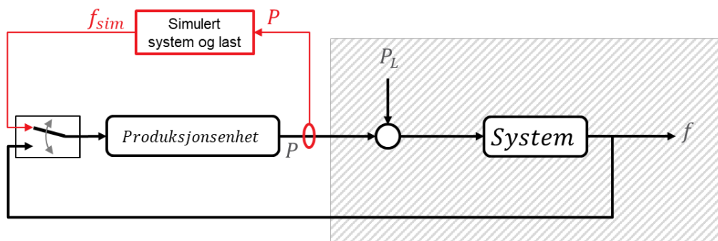
FIGUR 13-21: PRINSIPIELL VIRKEMÅTE FOR EN SIMULERT SEPARATCHRIFT VED HJELP AV HARDWARE IN THE LOOP (HWIL)
