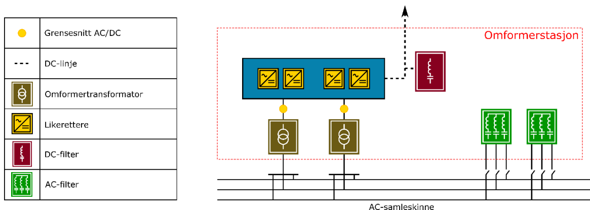
FIGUR 17-1: EKSEMPEL PÅ KOMPONENTER SOM KAN INNGÅ I EN OMFORMERSTASJON
