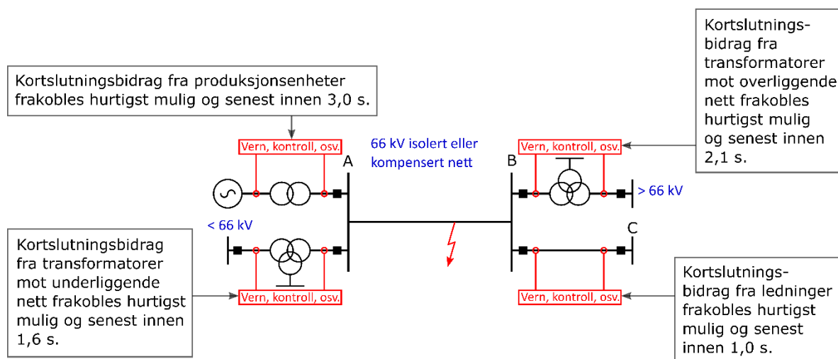
FIGUR 7-5: FRAKOBLING AV FEIL VED VERNSYSTEM- ELLER EFFEKTBYTERSVIKT
