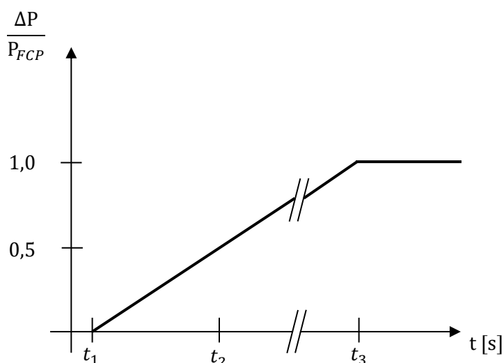
Figur 2 Effektrespons forbruk ved en stegforandring i frekvens. (Figur oppdatert)
