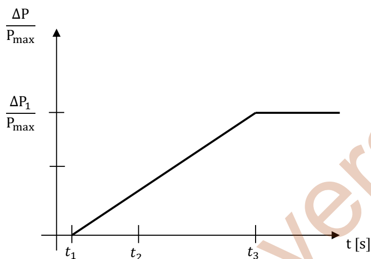
Figur 1 Effekterespons forbruk ved en stegforandring i frekvens.
