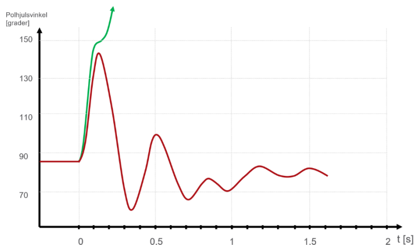
FIGUR 13-4: TYPISK TIDSFØRSLØP FOR ROTORVINKEL I TILKNYTNINGSPUNKT NÅR SYNKRONISME MOT NETTET BEHOLDSES (RØD) OG TAPES (GRØNN).
