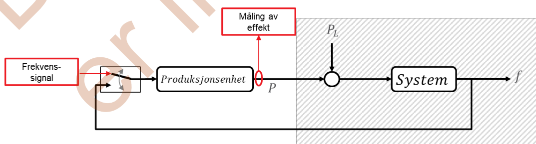
FIGUR 13-20: PRINSIPELL VIRKEMÅTE FOR EKSTERNT EKSTASJON AV TURBINREGULATOR
