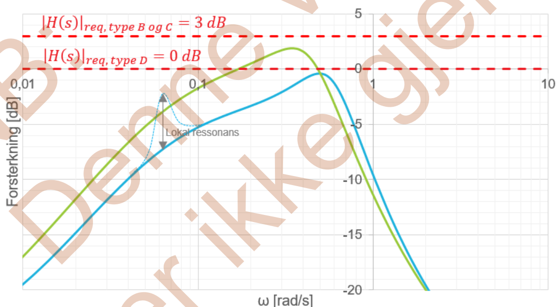
FIGUR 13-11: FREKVENSRRESPONS ILLUSTRERT I FREKVENSPANET VED 1 % LASTPÅSLAG REFERERT P_{maks} , VED P_{sett} = 0,85 \cdot P_{maks} OG 2 % STATISK. DE RØDE STIPLEDE LINJENE REPRERENTERER KRAVENE TIL MAKSIMALT TRANSIENT FREKVENSAVVIK. GRØNN (TYPE B OG C) OG BLÅ KURVER (TYPE D) ER EKSEMPLER PÅ FREKVENSFORLØP ETTER ET LASTSPRANG PÅ EGET OHMSK NETT.
