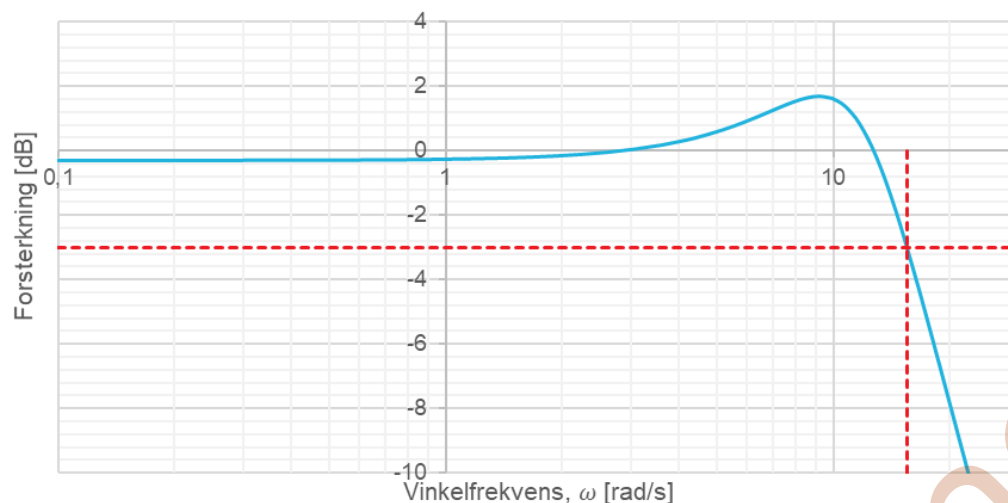
FIGUR 13-17: ILLUSTRASJON AV LUKKET SLØYFE-FORSTERKNING (BLÅ) FOR MAGNETISERINGSUTSTYR, MED BÅNDBREDEDE ILLUSTRERT (RØDSTIPILET)
