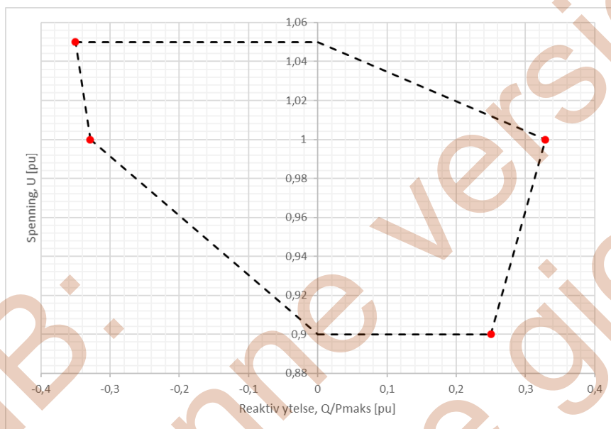
FIGUR 16-3: REAKTIV YTELSE FOR EN KRAFTPARK VED VARIERENDE SPENNING, I U - Q/P_{maks} -PROFIL. RØDE PUNKTER ANGRIR VERDIENE SOM SKAL DOKUMENTERES.
