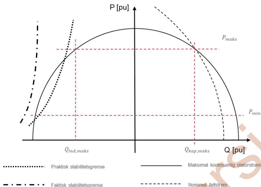
FIGUR 12-7: DRIFSDIAGRAMMET TIL EN TYPISK SYNKRONGENERATOR
