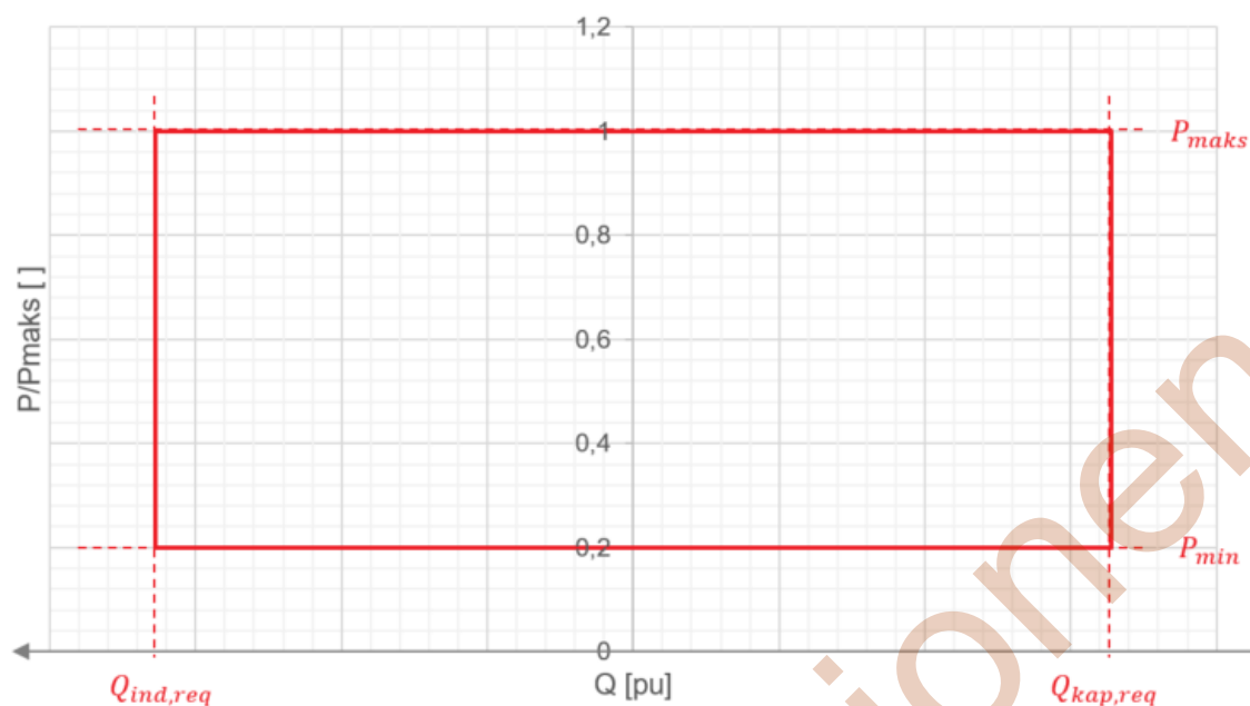
FIGUR 14-8: KRAV TIL MINIMUM REAKTIV YTELSE VED VARIERENDE AKTIV EFFEKT, P - Q/P_{maks} -DIAGRAM. Q_{kap,req} OG Q_{ind,req} ER GITT AV KAPITTEL 14.5.1.
