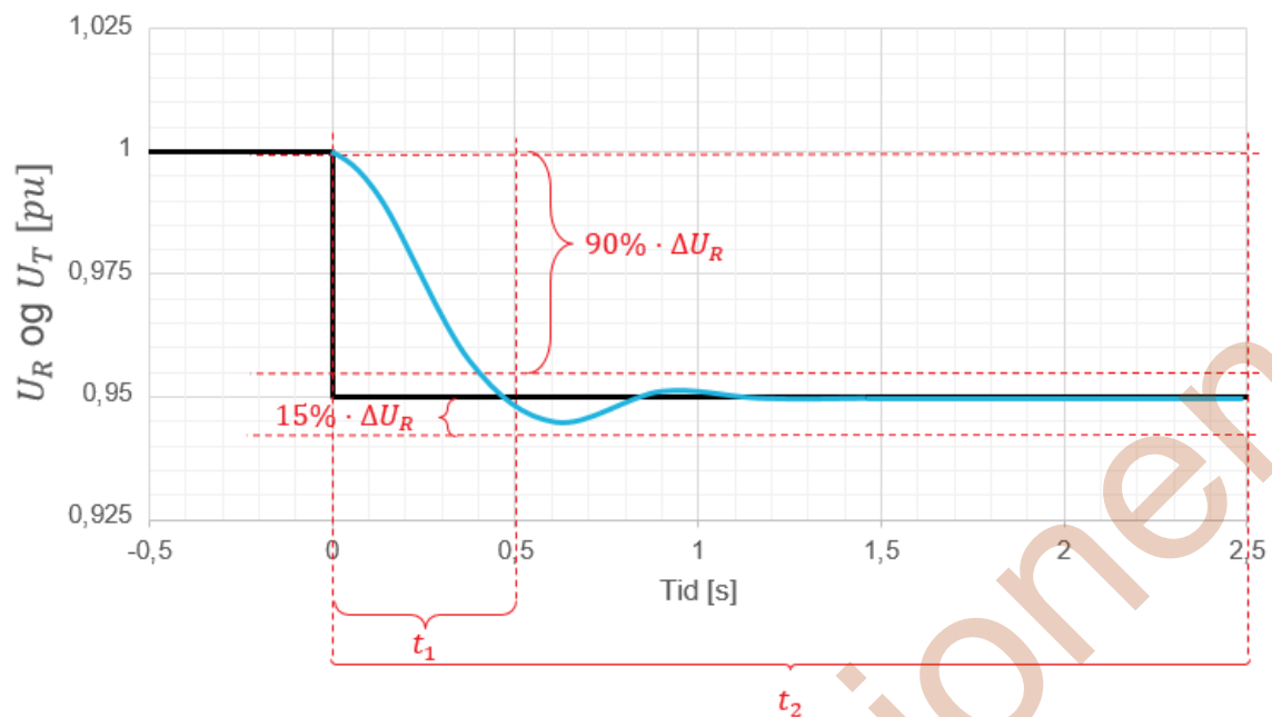
FIGUR 13-33: ILLUSTRASJON AV PRØVER FOR DOKUMENTASJON AV KRAV TIL UTREGULERINGSTID AV SPENNINGREFERANSESTEG I NEGATIV RETNING FOR MAGNETISERINGSUTSTYR MED ÅPNE GENERATORKLEMMER FOR SYNKRONE PRODUKSJONSENHETER.
