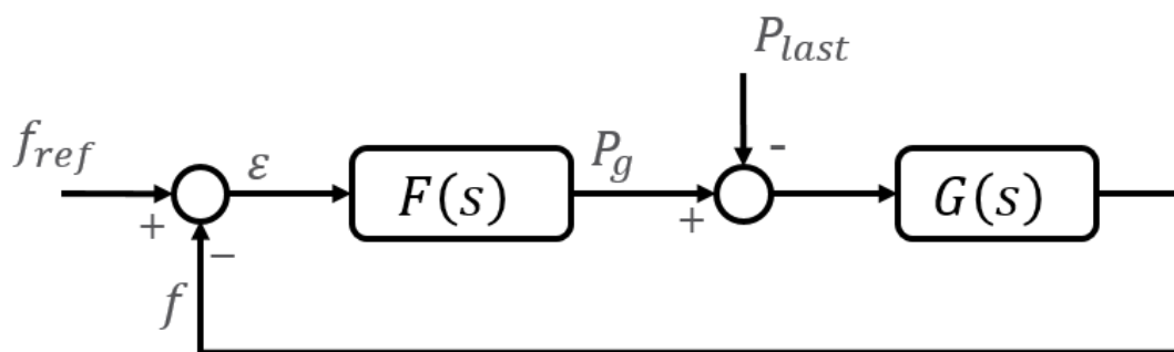
FIGUR 13-12: LUKKET SLØYFE
