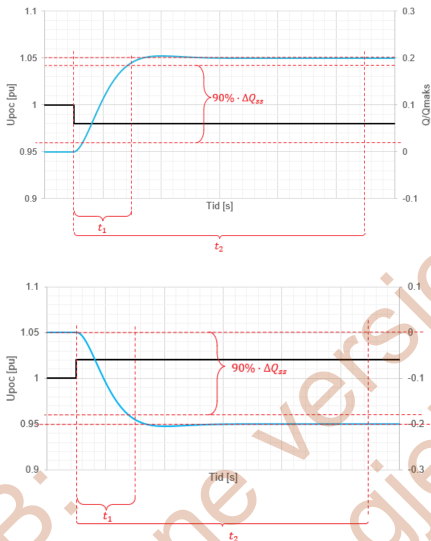
FIGUR 18-6: REAKTIV EFFEKTRESPONS VED STEGISVIS ENDRING I SPENNING PÅ HHV \pm 2\% . KRAV ER MARKERT I RØDSTIPLEDE LINJER
