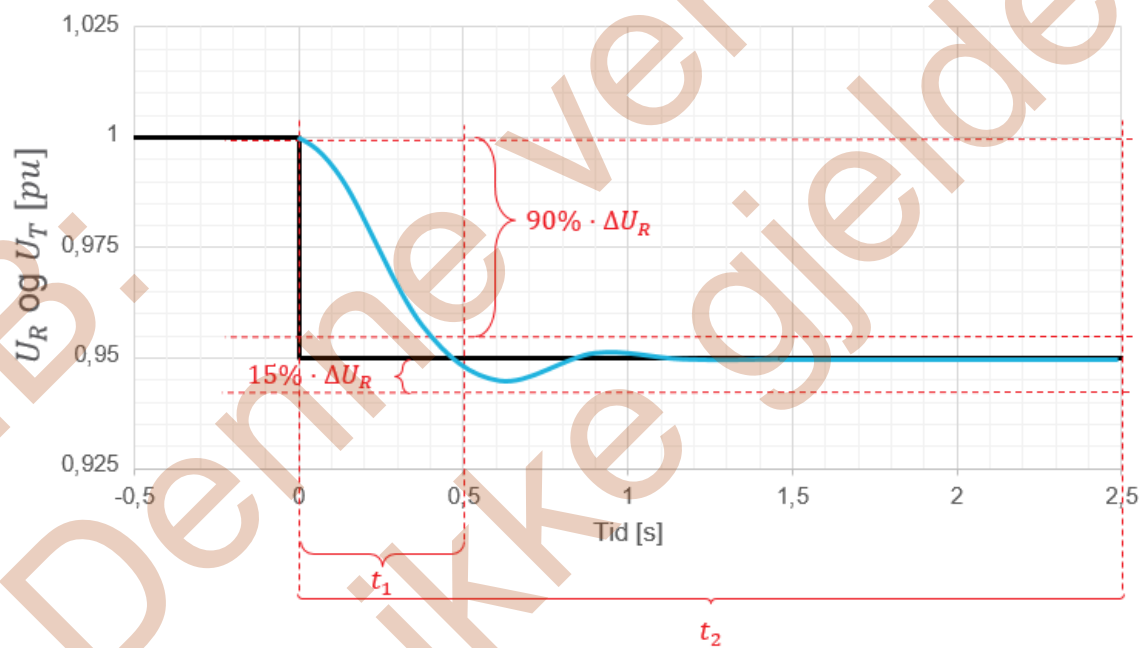
FIGUR 13-16: ILLUSTRASJON AV KRAV TIL UTREGULERINGSTID AV SPENNINGSPREFERANSESTEG I NEGATIV RETNING FOR MAGNETISERINGSUTSTYR I LUKKET SLØYFE MED ÅPEN EFFEKTBYTER FOR SYNKRONE PRODUKSJONSENHETER.
