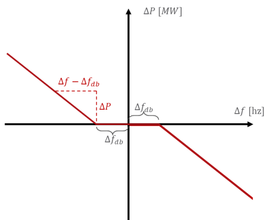
FIGUR 12-4: REGULATORRESPONS SOM FUNKSJON AV FREKVENSI I FREKVENSRULERINGSMODUS FOR SYNKRONE PRODUKSJONSENHETER.
