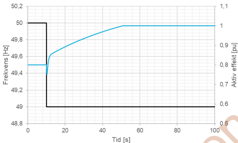
FIGUR 13-28: ILLUSTRASJON AV PRØVE AV AKTIV EFFEKTRESPONS (BLÅ) VED DETEKSIJON AV SEPARATDRIFT VED HØY FREKVENSENDRINGSNØYSE (ROCOF) VED PÅTRYKKET FREKVENSRAMPE (SORT).
