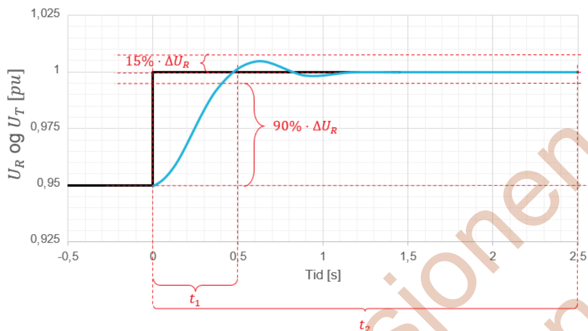
FIGUR 12-8: ILLUSTRASJON AV KRAV TIL UTREGULERINGSTID AV SPENNINGSPREFERANSESTEG I POSITIV RETNING FOR MAGNETISERINGSUTSTYR I LUKKET SLØYFE MED ÅPEN EFFEKTBRUYTER FOR SYNKRONE PRODUKSJONSENHETER.
