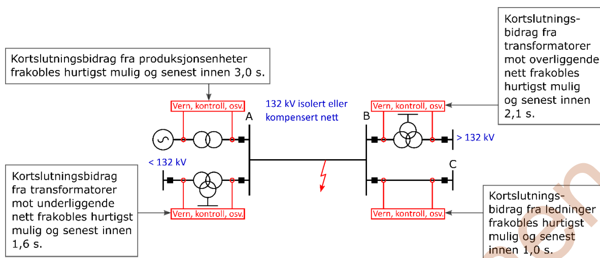
FIGUR 7-3: FRAKOBLING AV FEIL VED VERNSYSTEM- ELLER EFFEKTBYTTERSVIKT
