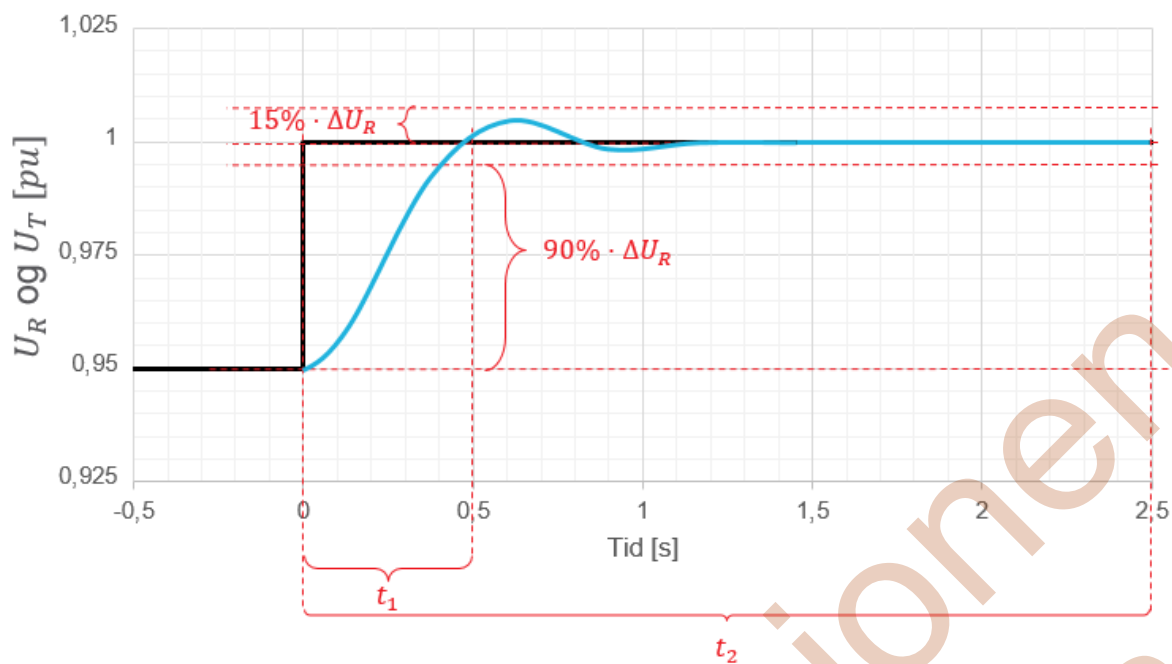
FIGUR 13-15: ILLUSTRASJON AV KRAV TIL UTREGULERINGSTID AV SPENNINGSPREFERANSESTEG I POSITIV RETNING FOR MAGNETISERINGSUTSTYR I LUKKET SLØYFE MED ÅPEN EFFEKTBYTER FOR SYNKRONE PRODUKSJONSENHETER.
