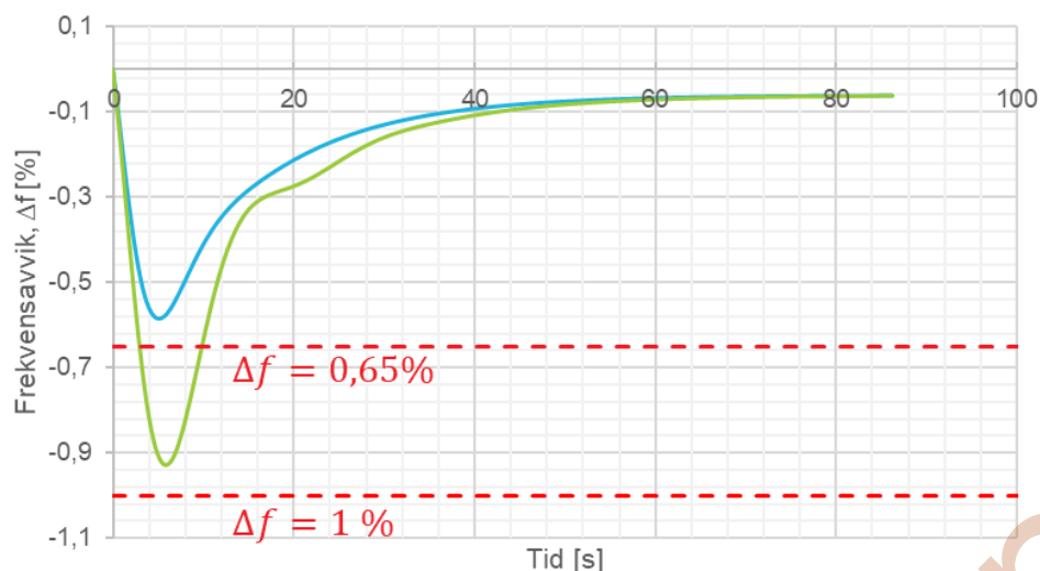
FIGUR 13-10: FREKVENSRRESPONS I TIDSPLANET VED 1 % LASTPÅSLAG REFERERT P_{maks} , VED P_{sett} = 85\% \cdot P_{maks} OG 2 % STATISK. DE RØDE STIPLEDE LINJENE REPRERENTERER KRAVENE TIL MAKSIMALT TRANSIENT FREKVENSAVVIK. GRØNN (TYPE B OG C) OG BLÅ KURVER (TYPE D) ER EKSEMPLER PÅ FREKVENSFORLØP ETTER ET LASTSPRANG PÅ EGET OHMSK NETT.
