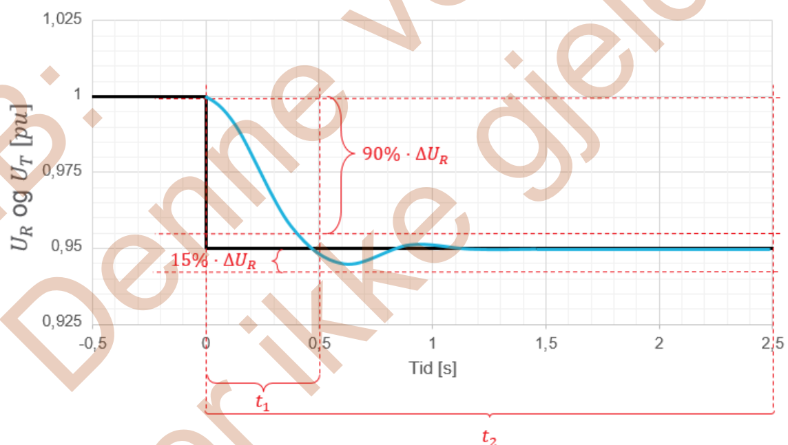
FIGUR 12-9: ILLUSTRASJON AV KRAV TIL UTREGULERINGSTID AV SPENNINGSPREFERANSESTEG I NEGATIV RETNING FOR MAGNETISERINGSUTSTYR I LUKKET SLØYFE MED ÅPEN EFFEKTBRUYTER FOR SYNKRONE PRODUKSJONSENHETER.
