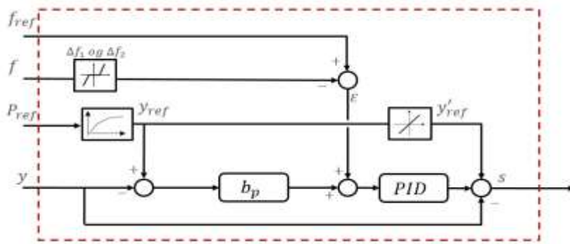
FIGUR 13-6: PRINSIPELL OPPBYGNING AV FREKVENREGULERING VED TILBAKEFØRING AV SERVOPOSISJON.
