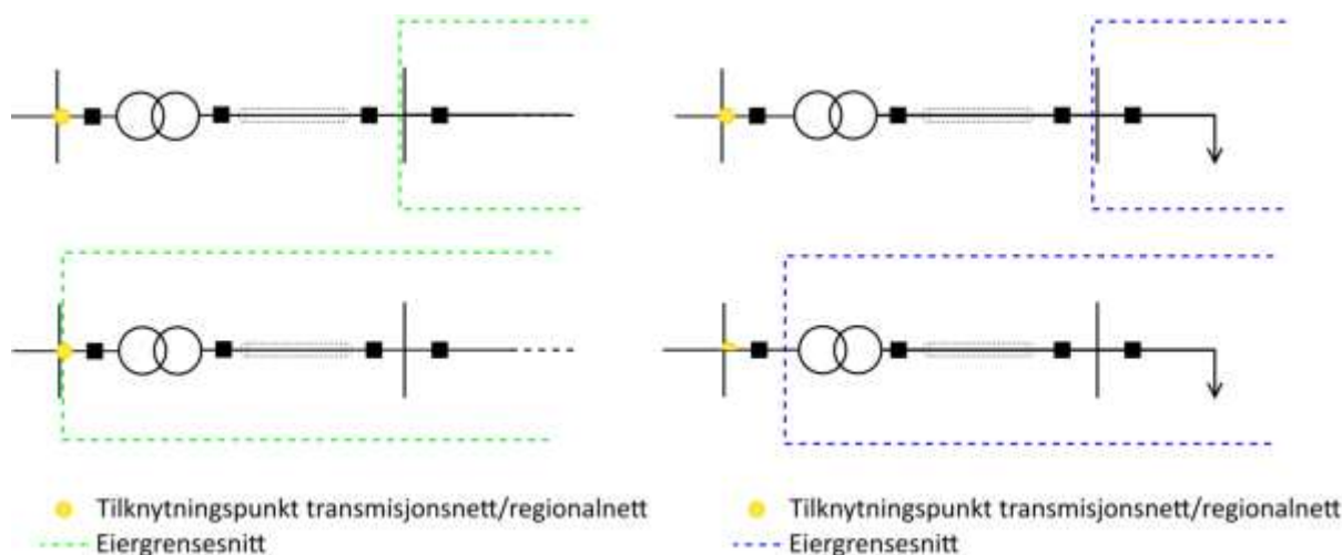
FIGUR 10-1 TILKOBLINGSPUNKT KAN VÆRE PÅ LAVSPENTSIDE AV TRANSFORMATOR TILKNYTTET REGIONAL- ELLER TRANSMISJONSNETT, VED EIERGRENSESNIITT. MENS DERSOM TILKNYTNING VIA TRANSFORMATOR, VIL REFERANSE FOR TILKNYTNINGSPUNKTET VIL ALLTID VÆRE PÅ HØYSPENTSIDE AV TRANSFORMATOREN.
