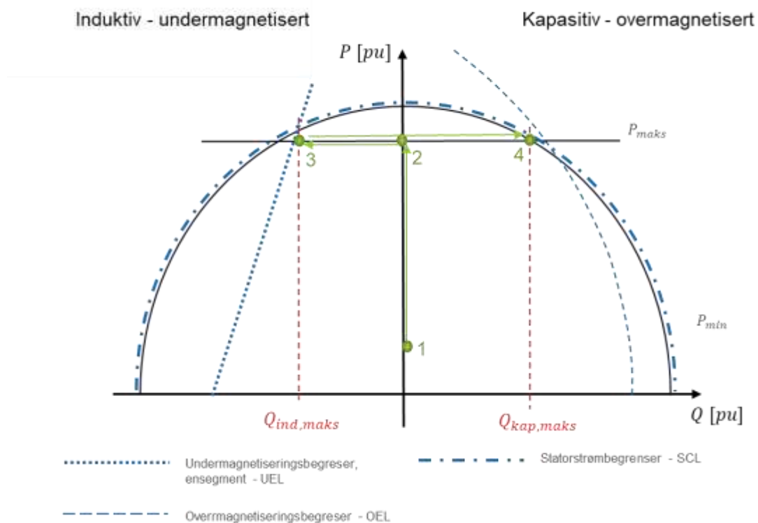
FIGUR 13-36: ILLUSTRASJON AV METODE FOR GJENNOMFØRING AV TEST AV REAKTIV YTELSE FOR SYNKRONE PRODUKSJONSENHETER. GRØNNE PUNKTER HENVISER TIL PUNKTLISTE OVER.
