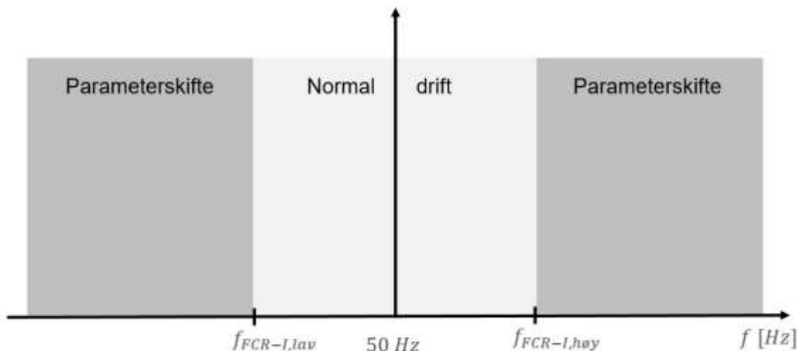
FIGUR 12-5: ILLUSTRASJON AV AUTOMATISK OG UFORSINKET AKTIVERING AV FCR-I VED KRITERIER FOR FCR-I.
