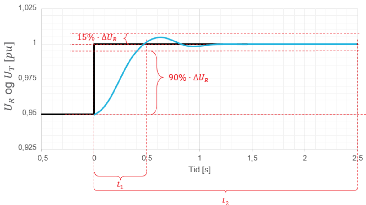
FIGUR 12-8: ILLUSTRASJON AV KRAV TIL UTREGULERINGSTID AV SPENNINGREFERANSESTEG I POSITIV RETNING FOR MAGNETISERINGSUTSTYR I LUKKET SLØYFE MED ÅPEN EFFEBTBRYTER FOR SYNKRONE PRODUKSJONSENHETER.
