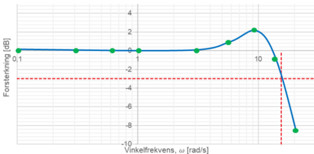
FIGUR 13-35: ILLUSTRASJON AV MAGNETISERINGSSYSTEMETS LUKKET SLØYFE-FORSTERKNING (BLÅ), MED BÅNDBREDDEN ILLUSTRERT (RØDSTIPELET). GRØNNE SIRKLER ILLUSTRERER DE TESTEDE PÅTRYKTE FREKVENSENE SOM ER TESTET.
