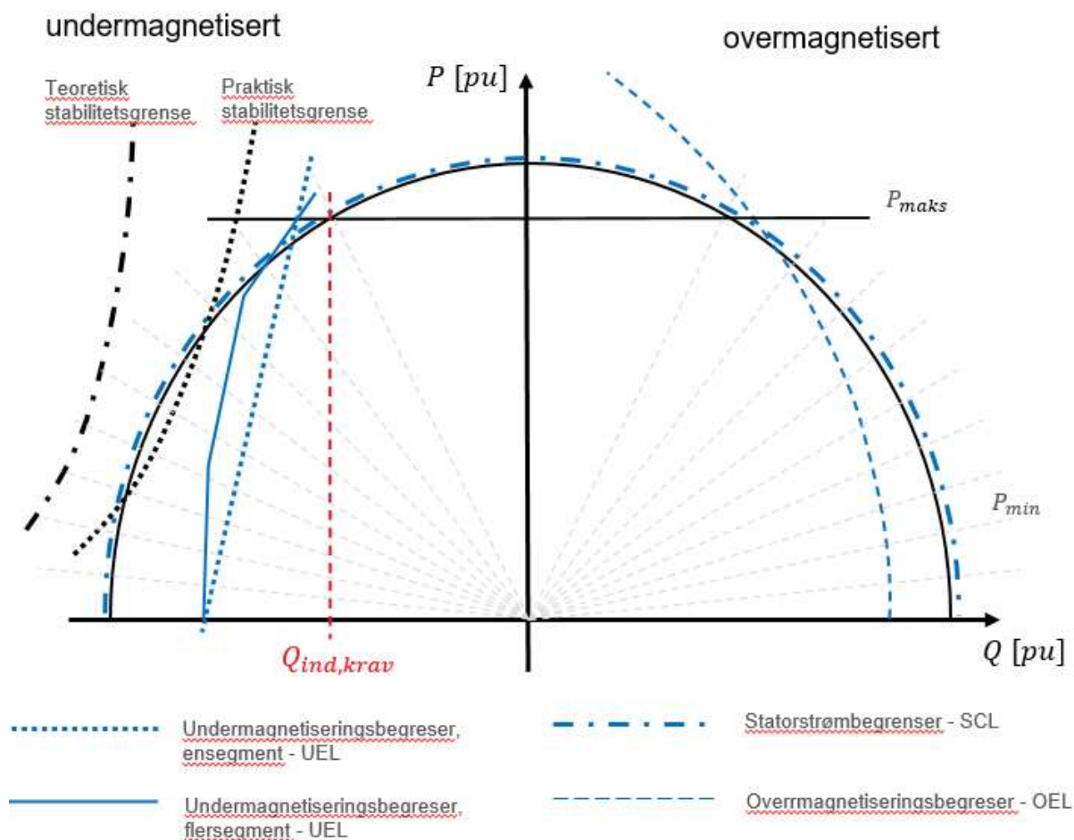
FIGUR 12-10: ILLUSTRASJON AV PRINSIPER FOR HVORDAN MAGNETISERINGSUTSTYRETS BEGRENSERE SKAL INNSTILLES.
