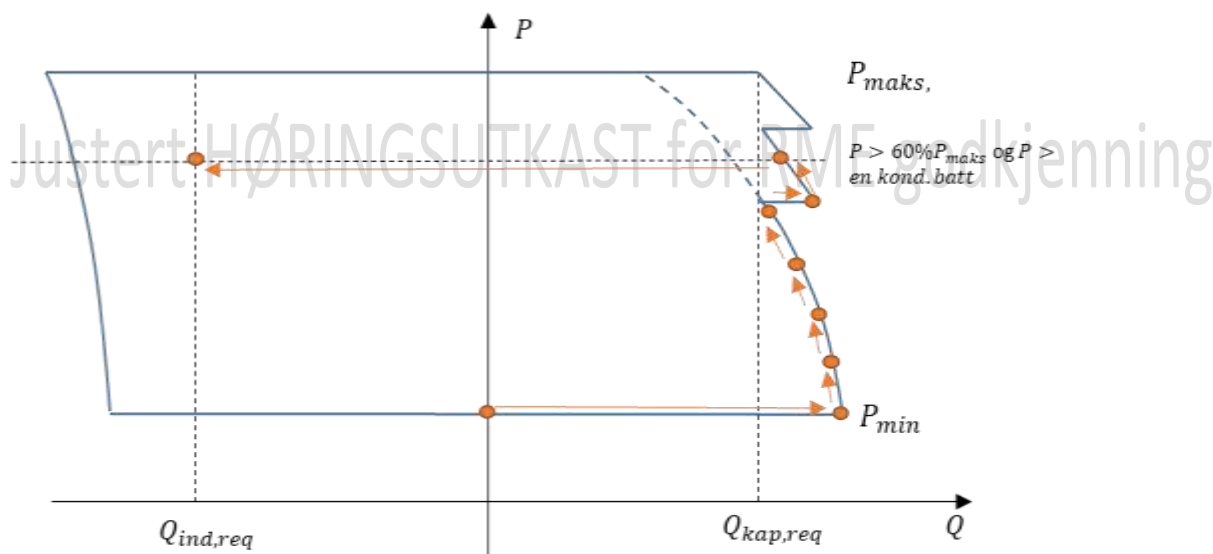
FIGUR 16-9: ILLUSTRASJON AV PROSEDYRE FOR DOKUMENTASJON AV REAKTIV YTELSE FOR EN KRAFTPARK, HER MED TO KONDENSATORBATTERIER I AUTOMATISKE STEG VED CA. P=50\% OG P=70\% . ORANGE PUNKTER MARKERER MÅLEPUNKTER SOM DOKUMENTERES. ALTERNATIVT LOGGES DET KONTINUERLIG VED ENDRING AV AKTIVE- OG REAKTIVE SETTPUNKTER.
