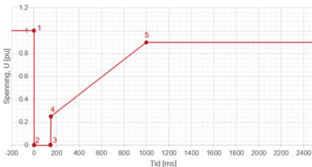
FIGUR 12-12: KRAV TIL FAULT RIDE THROUGH FOR TYPE D TILKNYTTET SPENNINGSNIVÅ \geq 110 kV. PRODUKSJONSENHETEN SKAL VÆRE TRANSIENT STABIL OG BEHOLDE SYNKRONISME FOR ALLE FEILFORLØP SOM GIR ET SPENNINGSFORLØP I TILKNYTNINGSPUNKTET SOM LIGGER OVER KURVEN.
