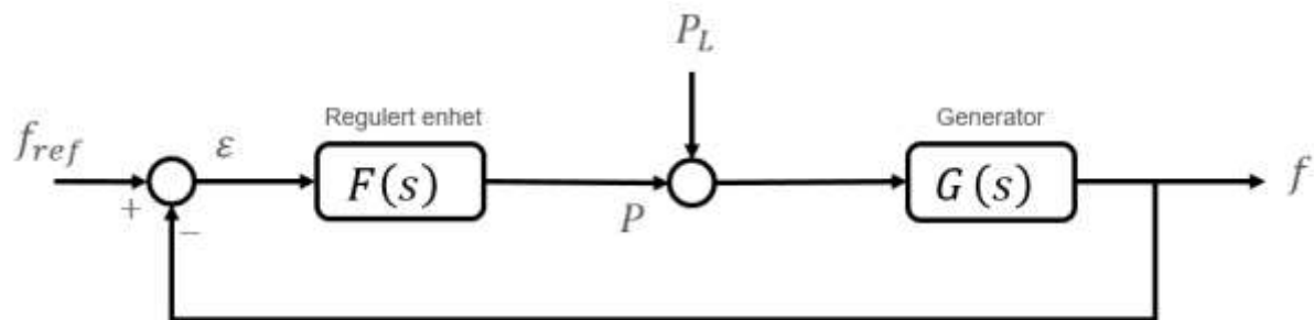
FIGUR 13-7: PRINSIPELL MODELLERING AV ET FREKVENREGULERT SYSTEM. F(S) ER DEN MATEMATISKE MODELLEN AV DEN REGULERTE ENHETEN (TURBINREGULATOR OG TURBINREGULERING). G(s) ER SYSTEMET.
