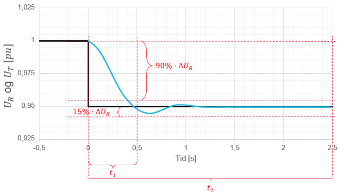
FIGUR 12-9: ILLUSTRASJON AV KRAV TIL UTREGULERINGSTID AV SPENNINGREFERANSESTEG I NEGATIV RETNING FOR MAGNETISERINGSUTSTYR I LUKKET SLØYFE MED ÅPEN EFFEBTBRYTER FOR SYNKRONE PRODUKSJONSENHETER.
