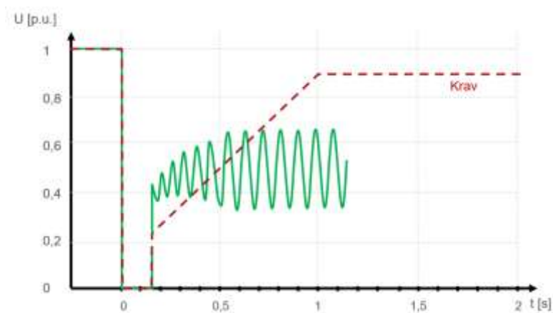
FIGUR 13-2: TYPISK TIDSFORLØP FOR SPENNING I TILKNYTNINGSPUNK NÅR SYNKRONISME MOT NETTET TAPES VED FEILKLARERINGSSTID > CCT, SELV OM SPENNINGEN LIGGER OVER KRAV-SPENNINGSPROFILEREN.
