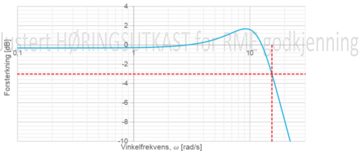
FIGUR 13-17: ILLUSTRASJON AV LUKKET SLØYFE-FORSTERKNING (BLÅ) FOR MAGNETISERINGSUTSTYR, MED BÅNDBREDDE ILLUSTRERT (RØDSTIPILET)
