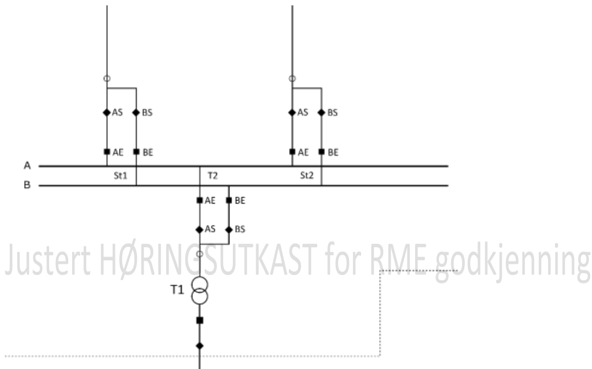
FIGUR 5-4: EKSEMPEL PÅ ENKELT BRYTERFELT PÅ SEKUNDÆRSIDE AV TRANSFORMATOR SOM TILKNYTTET EN ENKELT AVGANG
