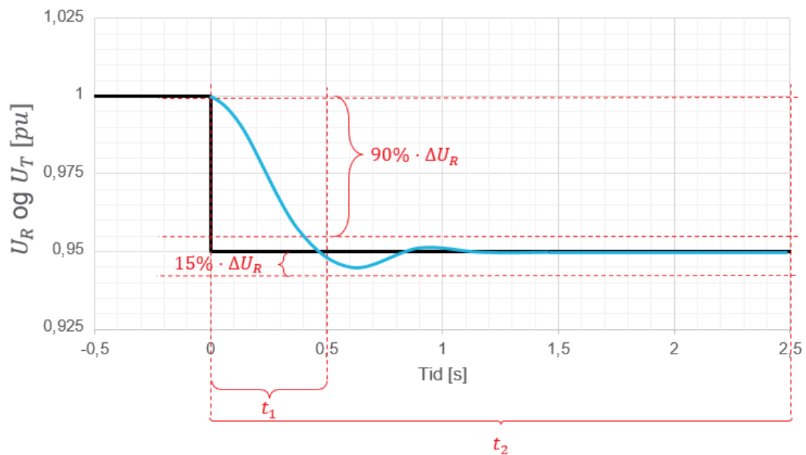
FIGUR 13-16: ILLUSTRASJON AV KRAV TIL UTREGULERINGSTID AV SPENNINGREFERANSESTEG I NEGATIV RETNING FOR MAGNETISERINGSUTSTYR I LUKKET SLØYFE MED ÅPEN EFFEKTBRUYER FOR SYNKRONE PRODUKSJONSENHETER.
