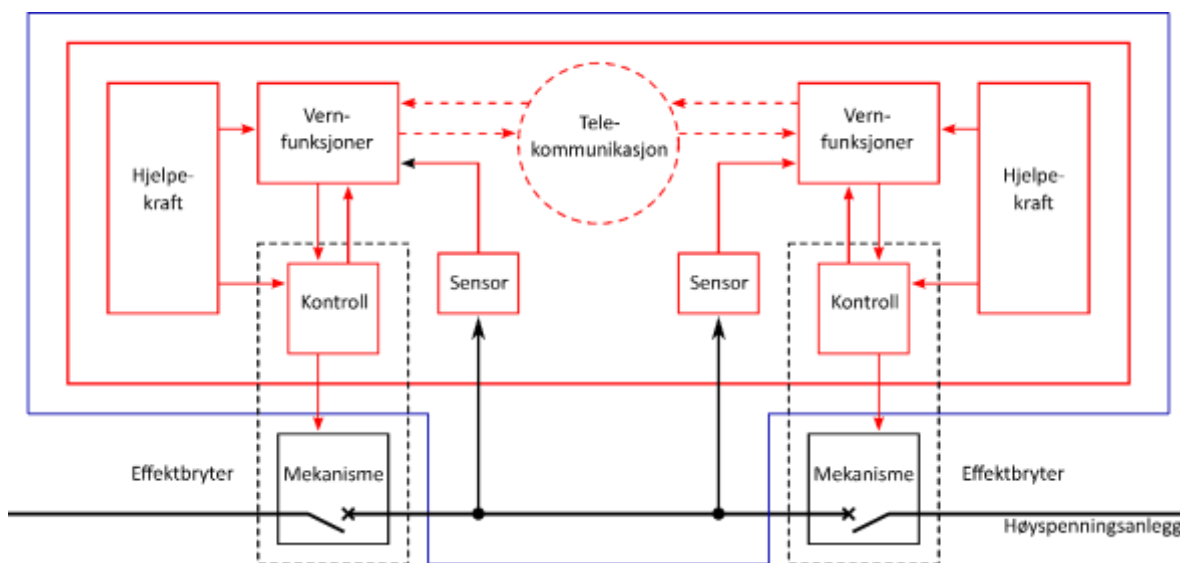
FIGUR 7-1: DEFINISJON FOR ENHET OG VERNSYSTEM
