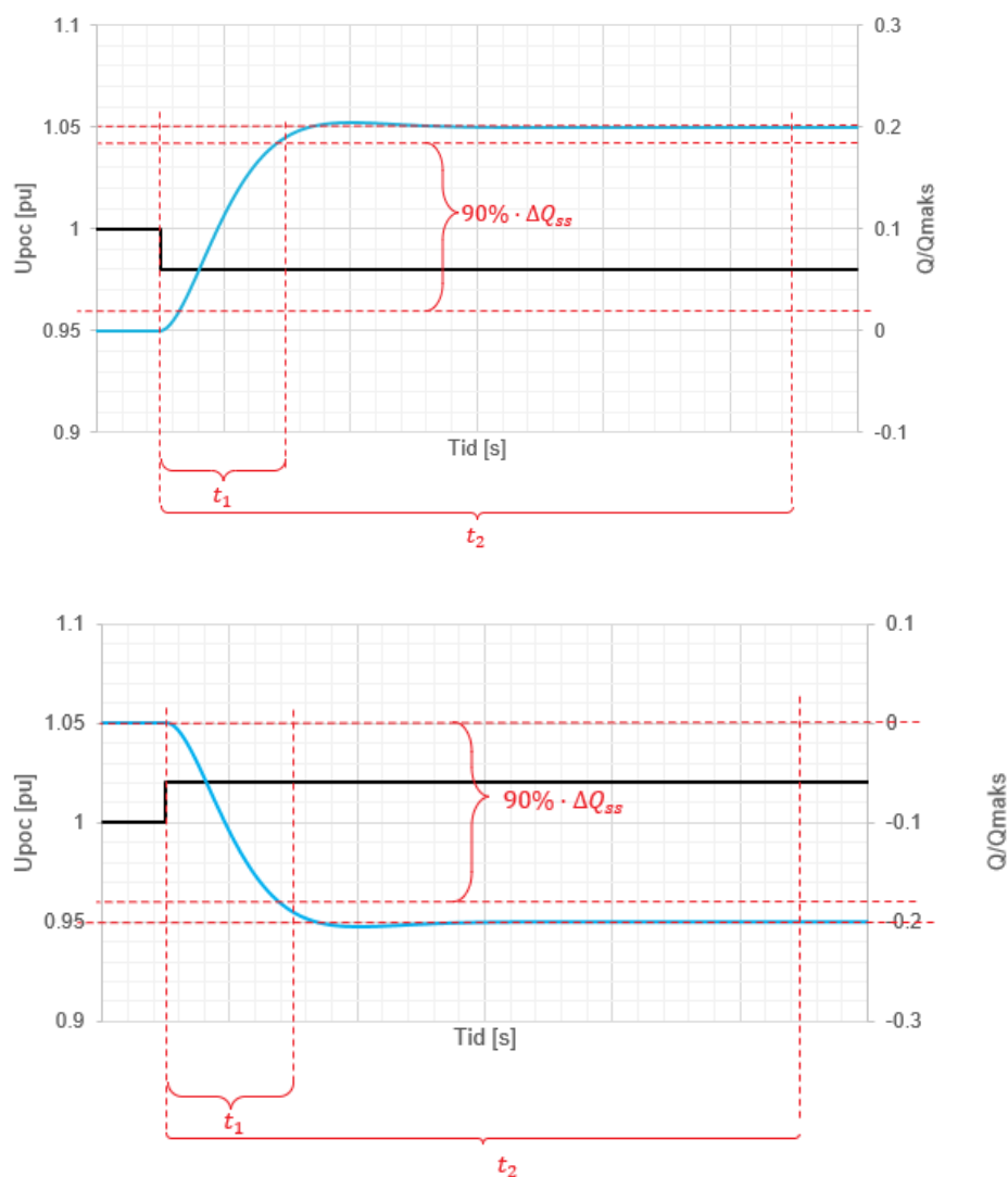
FIGUR 18-6: REAKTIV EFFEKTRRESPONS VED STEGVIS ENDRING I SPENNING PÅ HHV \pm 2\% . KRAV ER MARKERT I RØDSTIPELE LINJER
