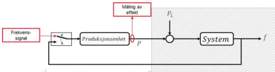
FIGUR 13-20: PRINSIPELL VIRKEMÅTE FOR EKSTERN EKSITASJON AV TURBINREGULATOR
