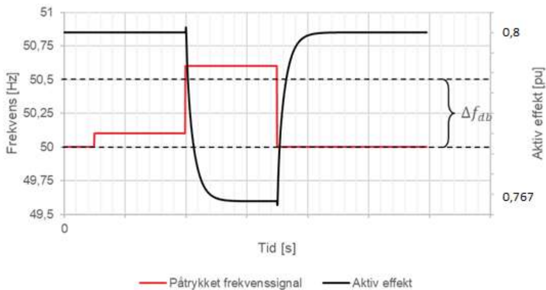
FIGUR 16-5: ILLUSTRASJON AV PRØVE FOR AKTIV EFFEKTRESPONS (SORT) VED PÅTRYKKET FREKVENNSTEG(RØD) MED AKTIVE DØDBÅND (SORT STIPILET LINJE).
