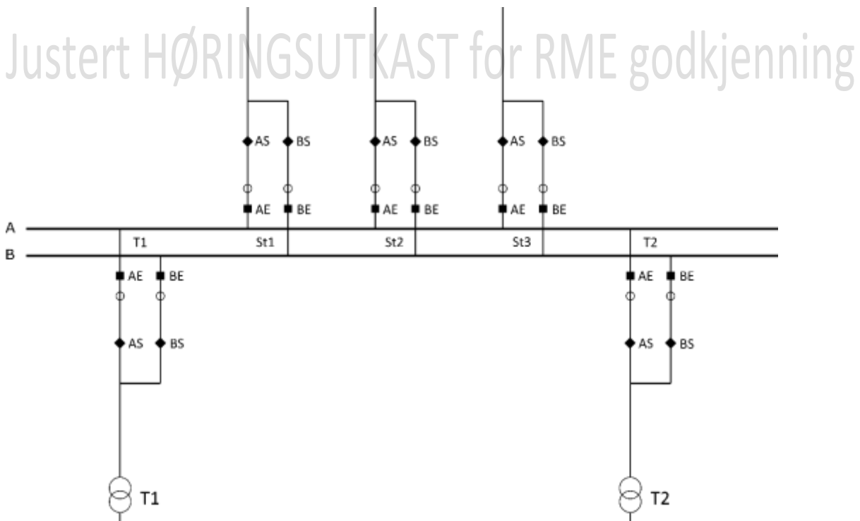
FIGUR 5-1: EKSEMPEL PÅ STASJONSLØSNING MED HØYESTE FLEKSIBILITET FOR LUFTISOLERT ANLEGG BASERT PÅ TO BRYTERE OG TO STRØMTRANSFORMATORER MED AB SKINNE.
