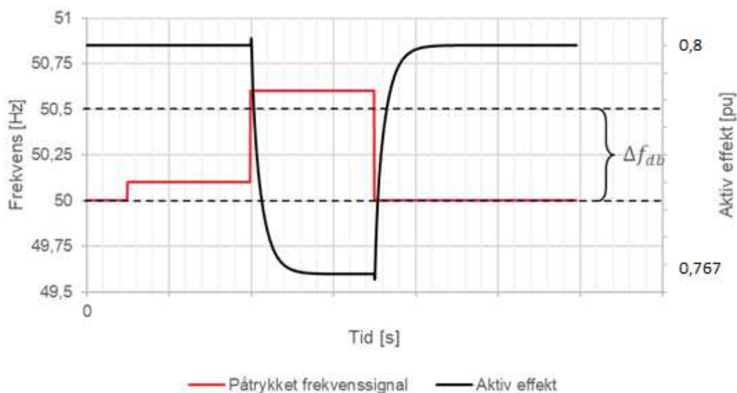
FIGUR 13-25: ILLUSTRASJON AV PRØVE FOR AKTIV EFFEKTRESPONS (SORT) VED PÅTRYKKET FREKVENSTEG (RØD) MED AKTIVE DØDBÅND (SORT STIPLLET LINJE).
