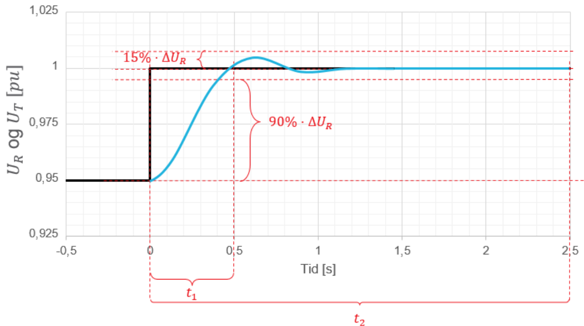
FIGUR 13-32: ILLUSTRASJON AV PRØVER FOR DOKUMENTASJON AV KRAV TIL UTREGULERINGS- TID AV SPENNINGREFERANSESTEG I POSITIV RETNING FOR MAGNETISERINGSUTSTYR MED ÅPNE GENERATORKLEMMER FOR SYNKRONE PRODUKSJONSENHETER.
