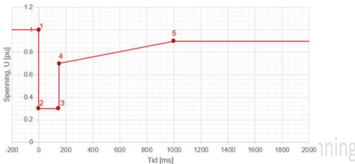
FIGUR 12-11: KRAV TIL FAULT RIDE THROUGH FOR TYPE A, B OG C, SAMT TYPE D TILKNYTTET SPENNINGSNIVÅ < 110 kV. PRODUKSJONSENHETEN SKAL VÆRE TRANSIENT STABIL OG BEHOLDE SYNKRONISME FOR ALLE FEILFORLØP SOM GIR EN SPENNING I TILKNYTNINGSPUNKTET SOM LIGGER OVER KURVEN.
