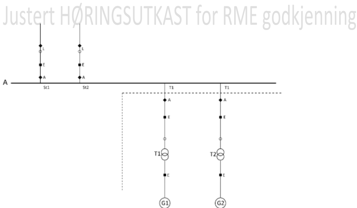
FIGUR 5-5: EKSEMPEL PÅ STASJONSANLEGG MED ENKEL FLEKSIBILITET
