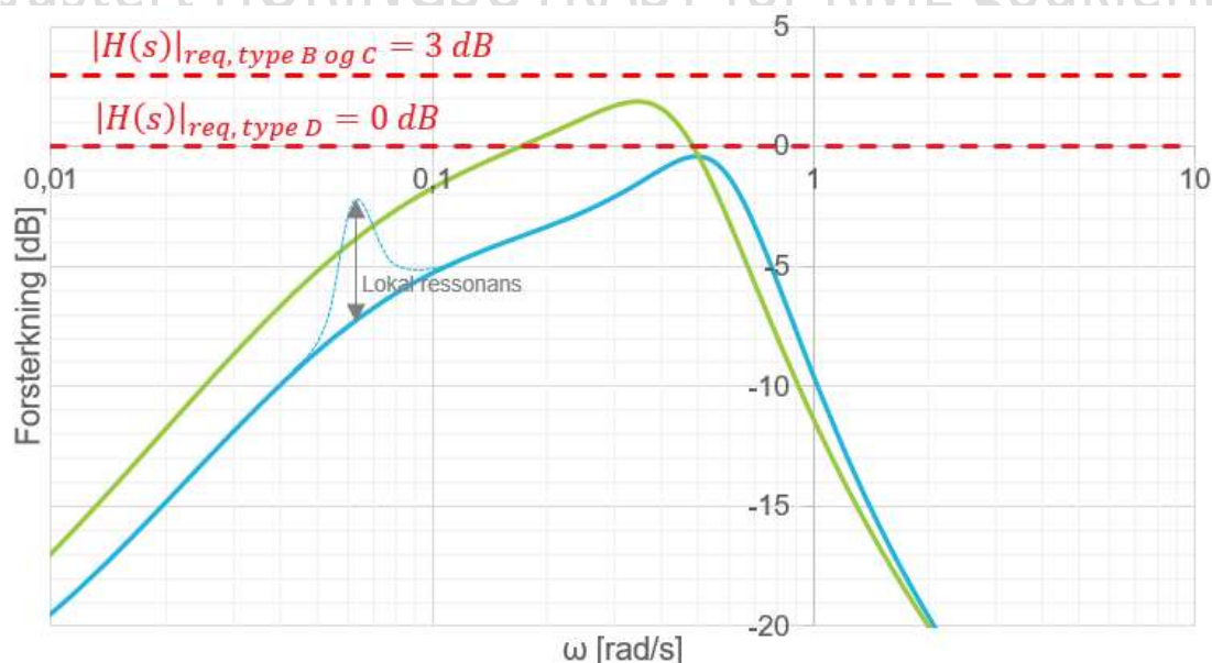
FIGUR 13-11: FREKVENSRSPONS ILLUSTRERT I FREKVENSPANET VED 1 % LASTPÅSLAG REFERERT P_{maks} , VED P_{sett} = 0,85 \cdot P_{maks} OG 2 % STATIKK. DE RØDE STIPLEDE LINJENE REPRERENTERER KRAVENE TIL MAKSIMALT TRANSIENT FREKVENSAVVIK. GRØNN (TYPE B OG C) OG BLÅ KURVER (TYPE D) ER EKSEMPLER PÅ FREKVENSFØRLØP ETTER ET LASTSPRANG PÅ EGET OHMSK NETT.
