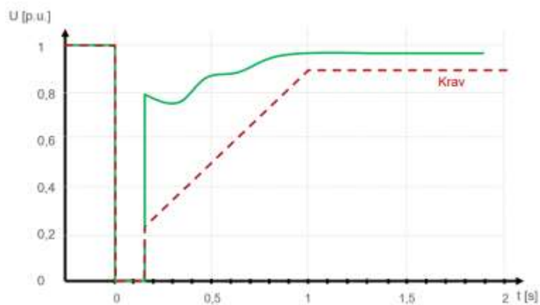
FIGUR 13-1: TYPISK TIDSFORLØP FOR SPENNING I TILKNYTNINGSPUNK NÅR SYNKRONISME MOT NETTET BEHOLDRES.
