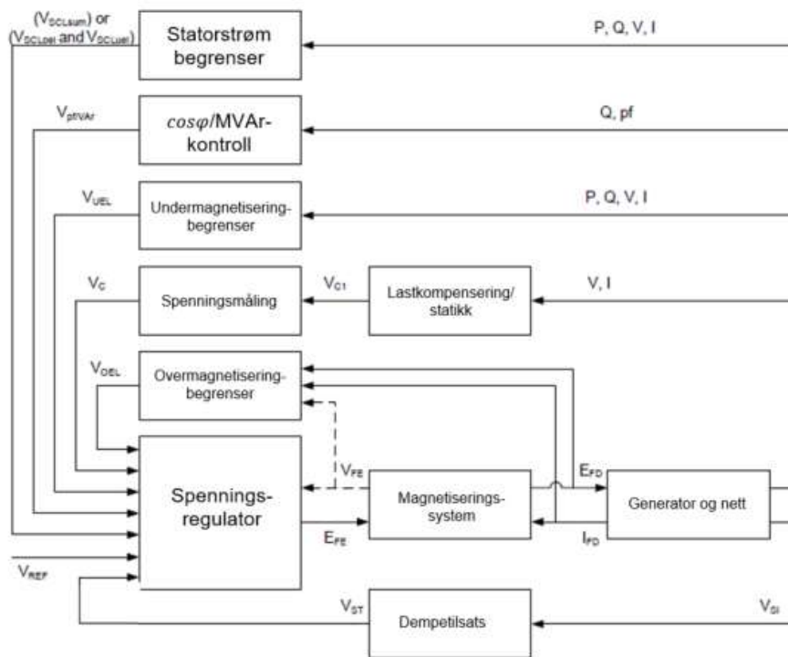
FIGUR 13-14: PRINSIPELL VIRKEMÅTE TIL SPENNINGREGULATOREN FOR EN SYNKRON PRODUKSJONSENHET [11]. NB; MERK AT BLOKDDIAGRAMMET KUN VISER SPENNINGSSINNGANG TIL DEMPETILSATS. DEMPETILSATS SKAL OGSÅ BENYTTE TURTALL IHT. KRAV I KAPITTEL 12.5.6.
