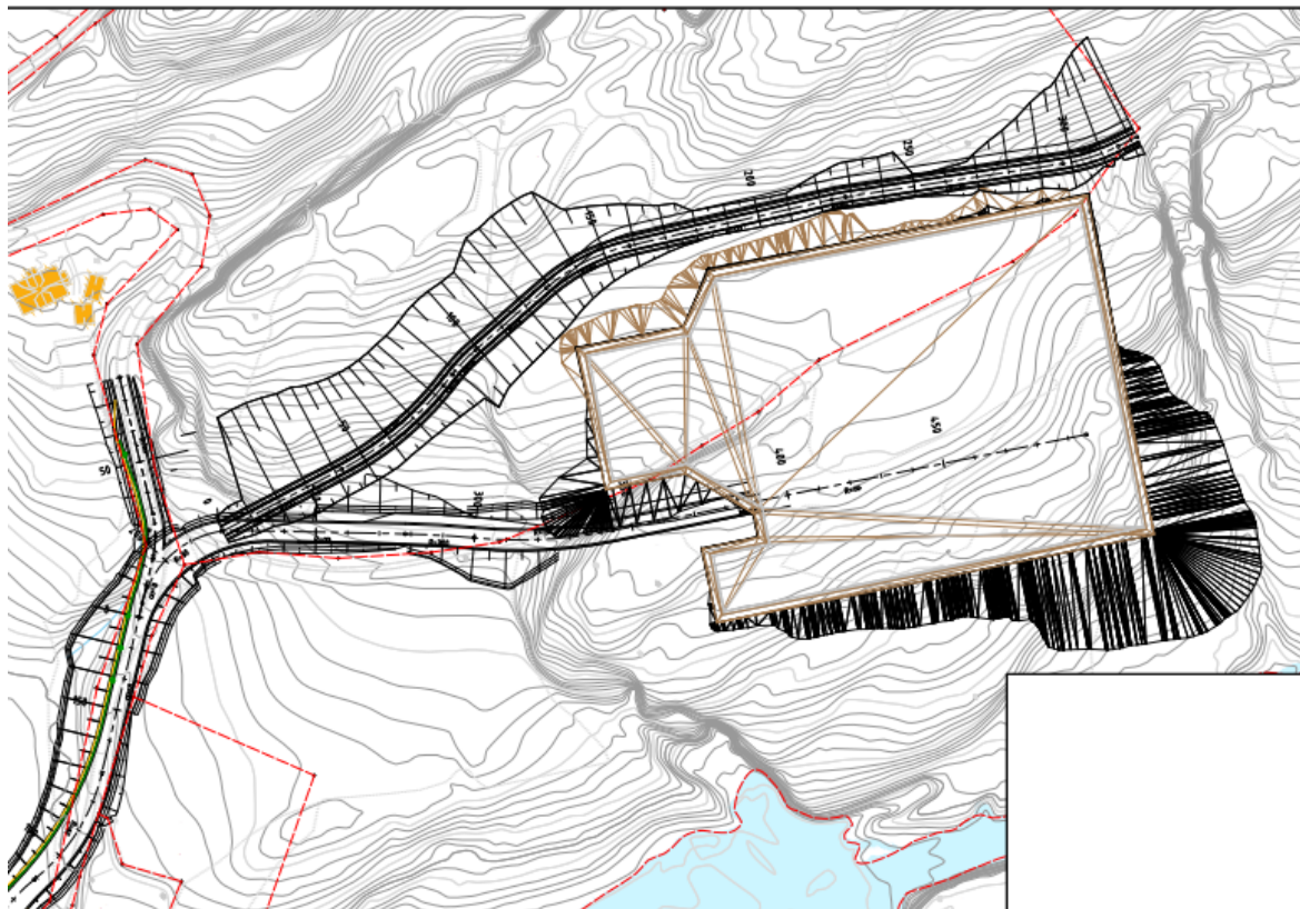
Figur 1 - også vist i komplett tegning vedlegg 1. Traktorvei med trasè fra konsesjonssøknad. Veiløsningen medfører skjæringer inn på landbruksareal og treffer eksisterende vei nord for stasjonen.
