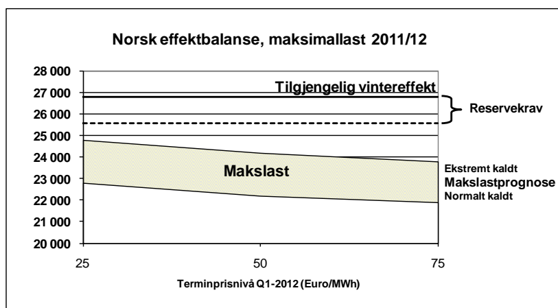
Figur 1 Norsk effektbalanse i maksimallastsituasjon 2011/12. Prognosert tilgjengelig vintereffekt og makslastforbruk.
