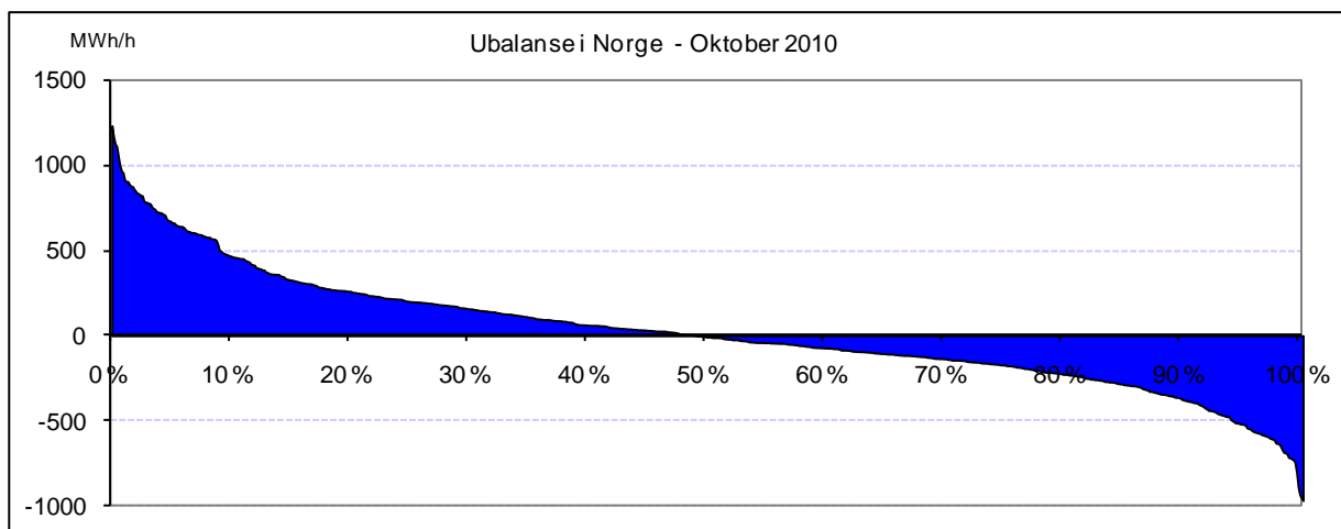
Figur 4: Varighetskurver for ubalanser i Norge i oktober 2010. Skjæringspunktet med x-aksen viser andel av tiden det var henholdsvis underskudd (pos) og overskudd (neg) av kraft.
