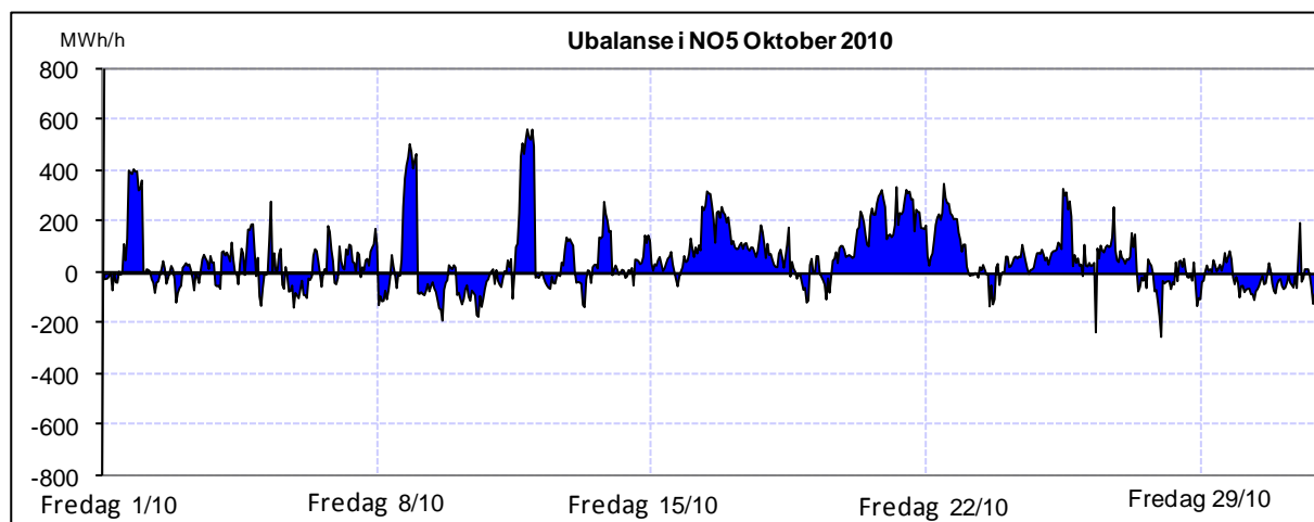
Figur 3: Ubalanser time for time i prisområdene NO1, NO2, NO3, NO4 og NO5, i oktober 2010. Ubalanser i det totale kraftsystemet innebærer at kraftflyten avviker i forhold til de planlagte verdier, og en positiv verdi indikerer et underskudd i prisområdet
