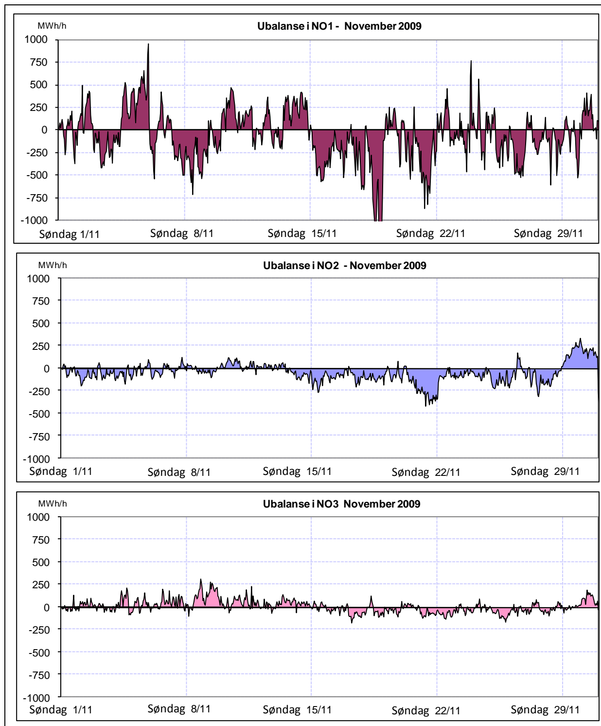
Figur 3: Ubalanser time for time i prisområdene NO1, NO2 og NO3, i november 2009. Ubalanser i det totale kraftsystemet innebærer at kraftflyten avviker i forhold til de planlagte verdier, og en positiv verdi indikerer et underskudd i prisområdet
