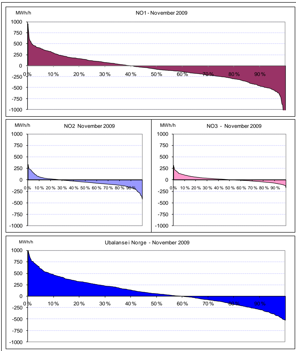
Figur 4: Varighetskurver for ubalanser i Norge i november 2009. Skjæringspunktet med x-aksen viser andel av tiden det var henholdsvis underskudd (pos) og overskudd (neg) av kraft.
