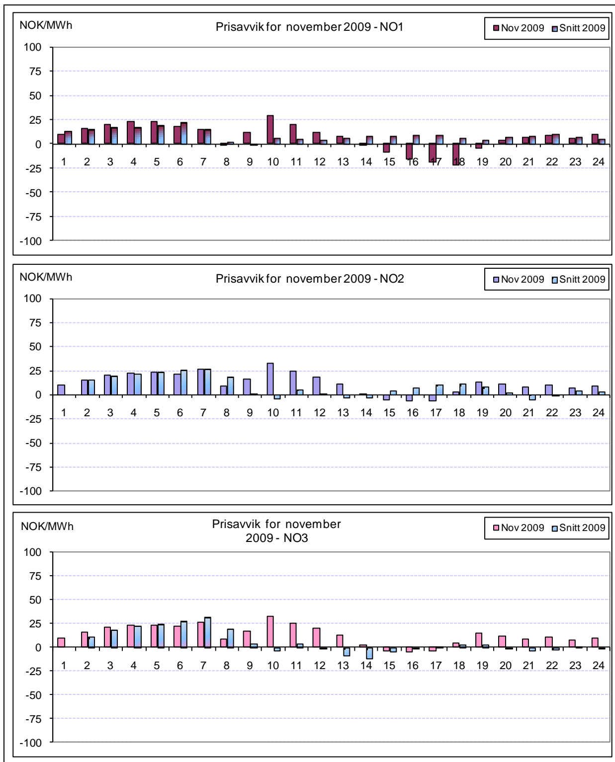
Figur 2: Prisavvik gjennom døgnet i november 2009 (Elspot – RK)
