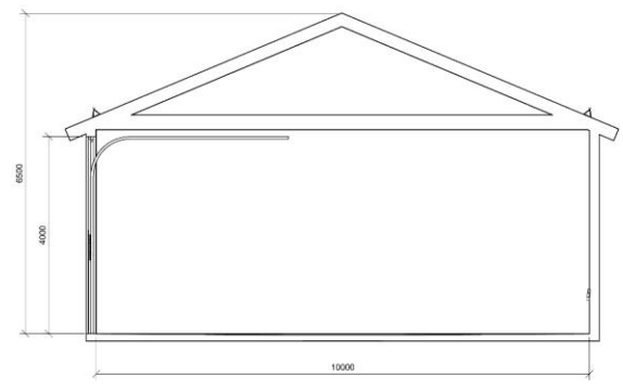
Snitt A 1 : 50
