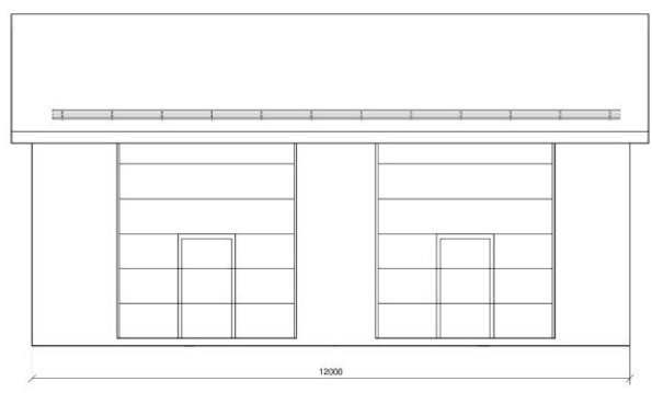
Fasade A 1 : 50
