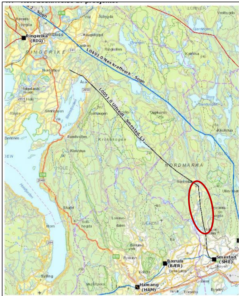
Figur 1: Oversiktskart over ledningen som skal rives vist med sort linje. Rød ellipse, påtegnet av oss, viser ca. strekning for ledningen som rives 1. januar 2021. Kilde: Statnetts MTA av 3. oktober 2021.
