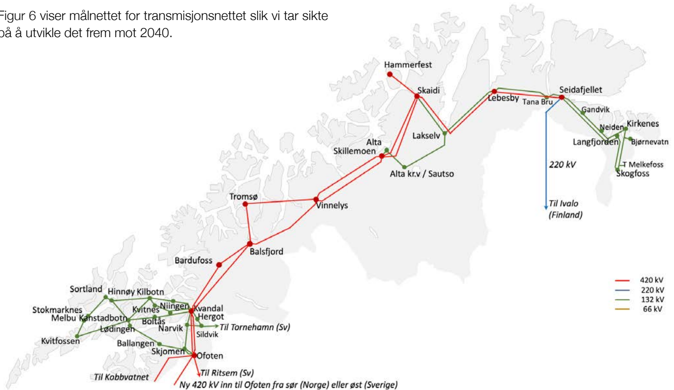
Figur 6: Målnett for transmisjonsnettet i område Nord, stadium 2040.
